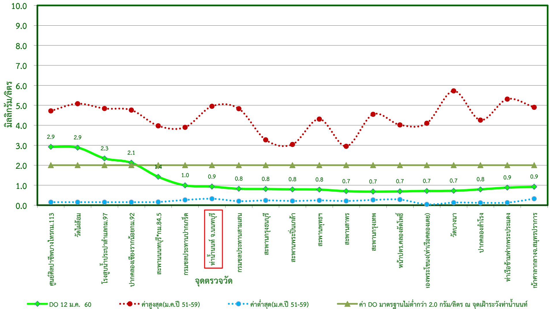
กราฟแสดงค่าออกซิเจนละลายน้ำในแม่น้ำเจ้าพระยาตามพระราชเสาวนีย์ฯ เมื่อวันที่ 12 มกราคม 2560
