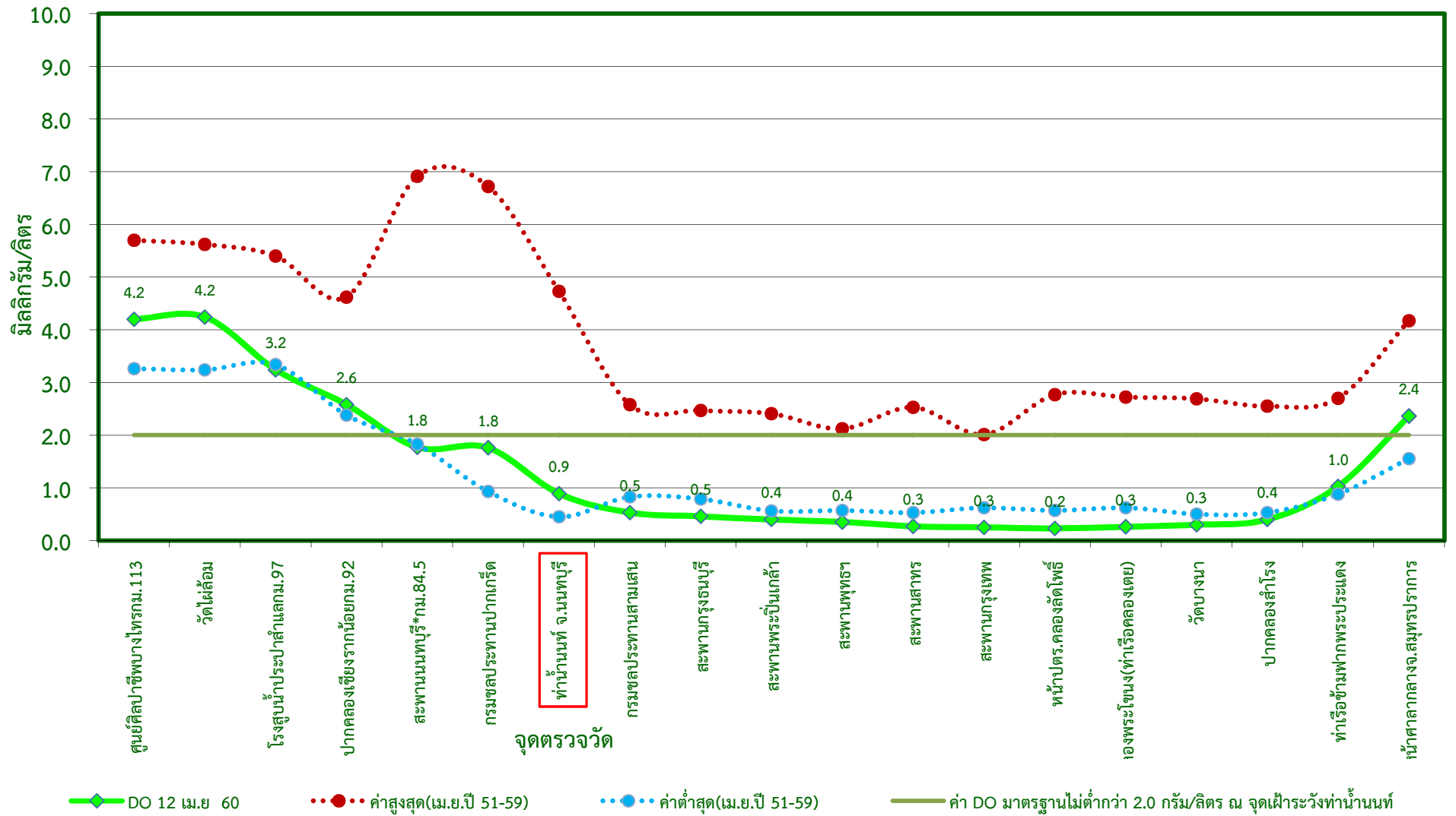
กราฟแสดงค่าออกซิเจนละลายน้ำในแม่น้ำเจ้าพระยาตามพระราชเสาวนีย์ฯ เมื่อวันที่ 12 เมษายน 2560
