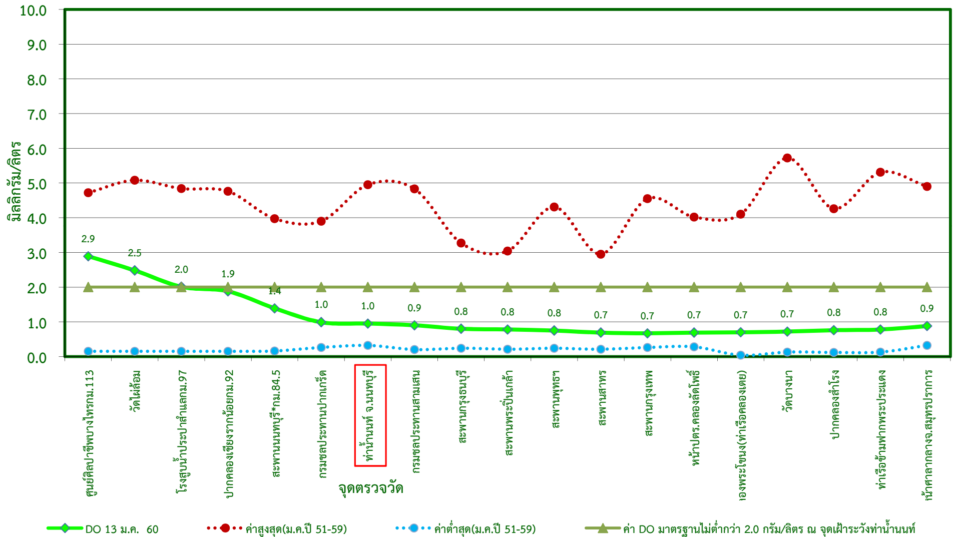
กราฟแสดงค่าออกซิเจนละลายน้ำในแม่น้ำเจ้าพระยาตามพระราชเสาวนีย์ฯ เมื่อวันที่ 13 มกราคม 2560
