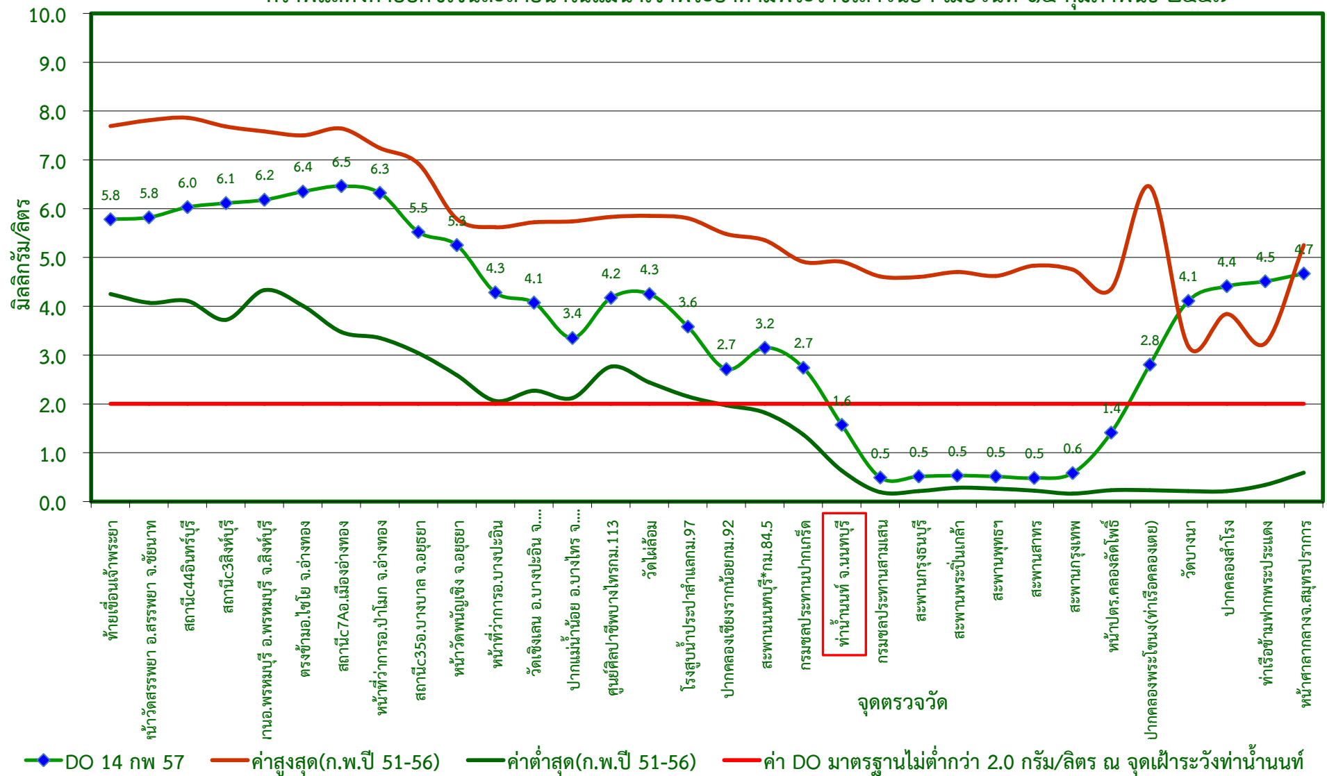
กราฟแสดงค่าออกซิเจนละลายน้ำในแม่น้ำเจ้าพระยาตามพระราชเสาวนีย์ฯ เมื่อวันที่ ๑๔ กุมภาพันธ์ ๒๕๕๗
