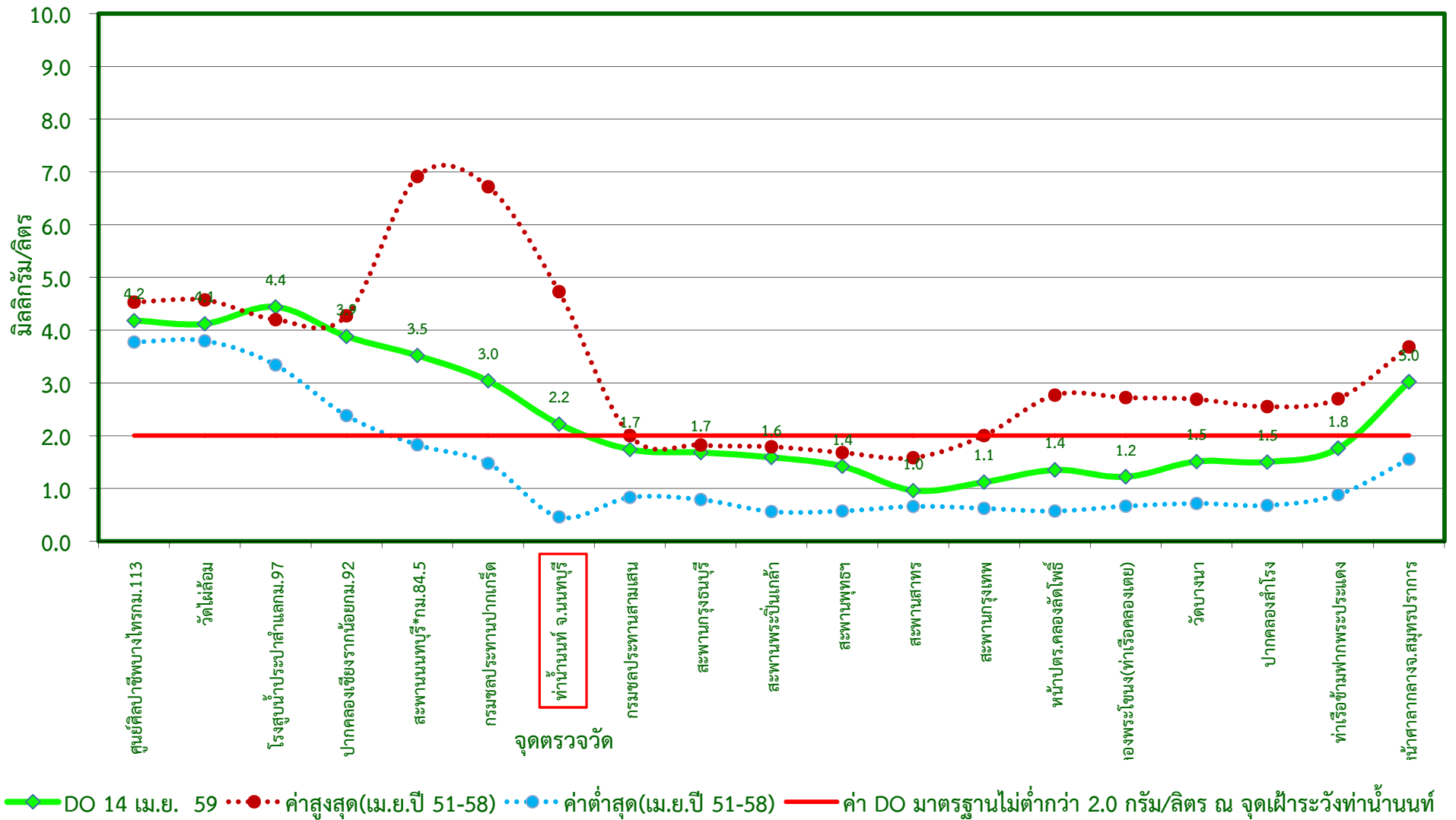
กราฟแสดงค่าออกซิเจนละลายน้ำในแม่น้ำเจ้าพระยาตามพระราชเสาวนีย์ฯ เมื่อวันที่ 14 เมษายน 2559
