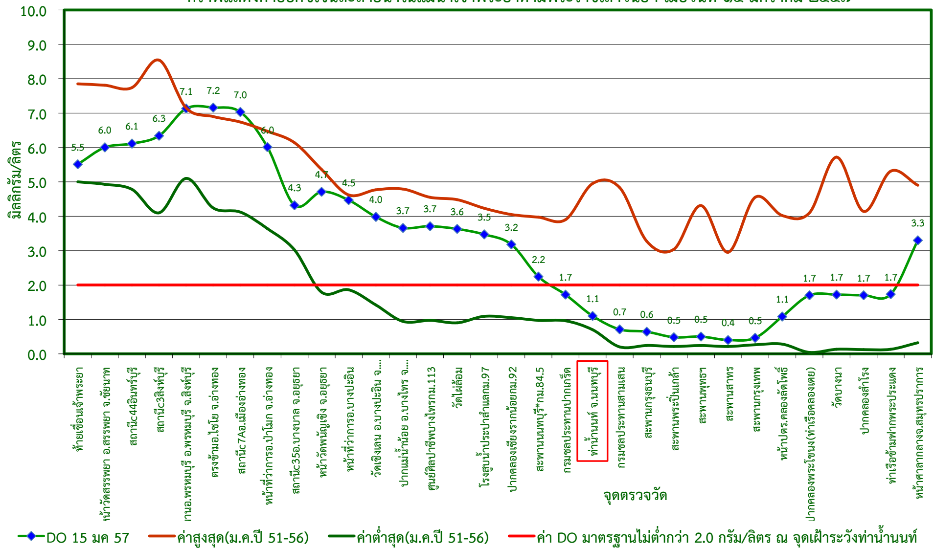
กราฟแสดงค่าออกซิเจนละลายน้ำในแม่น้ำเจ้าพระยาตามพระราชเสาวนีย์ฯ เมื่อวันที่ ๑๕ มกราคม ๒๕๕๗
