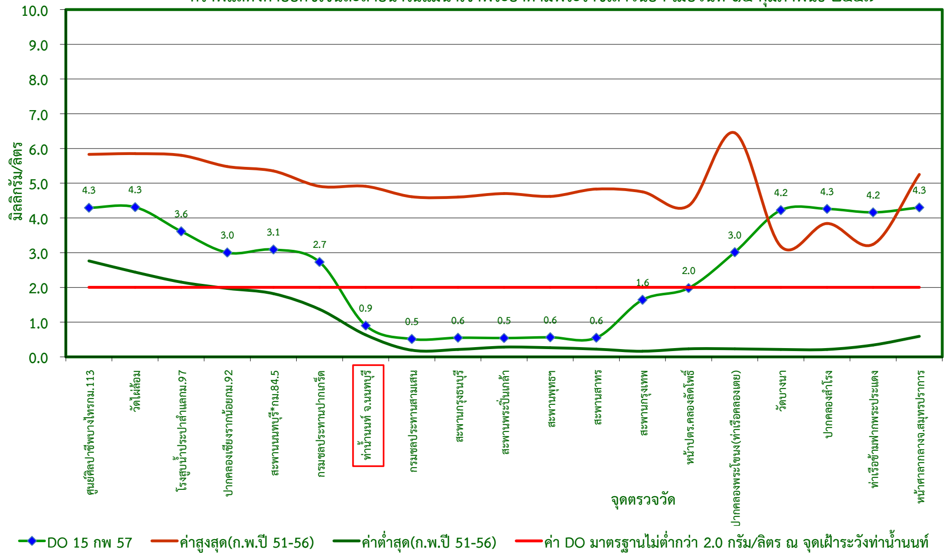
กราฟแสดงค่าออกซิเจนละลายน้ำในแม่น้ำเจ้าพระยาตามพระราชเสาวนีย์ฯ เมื่อวันที่ ๑๕ กุมภาพันธ์ ๒๕๕๗
