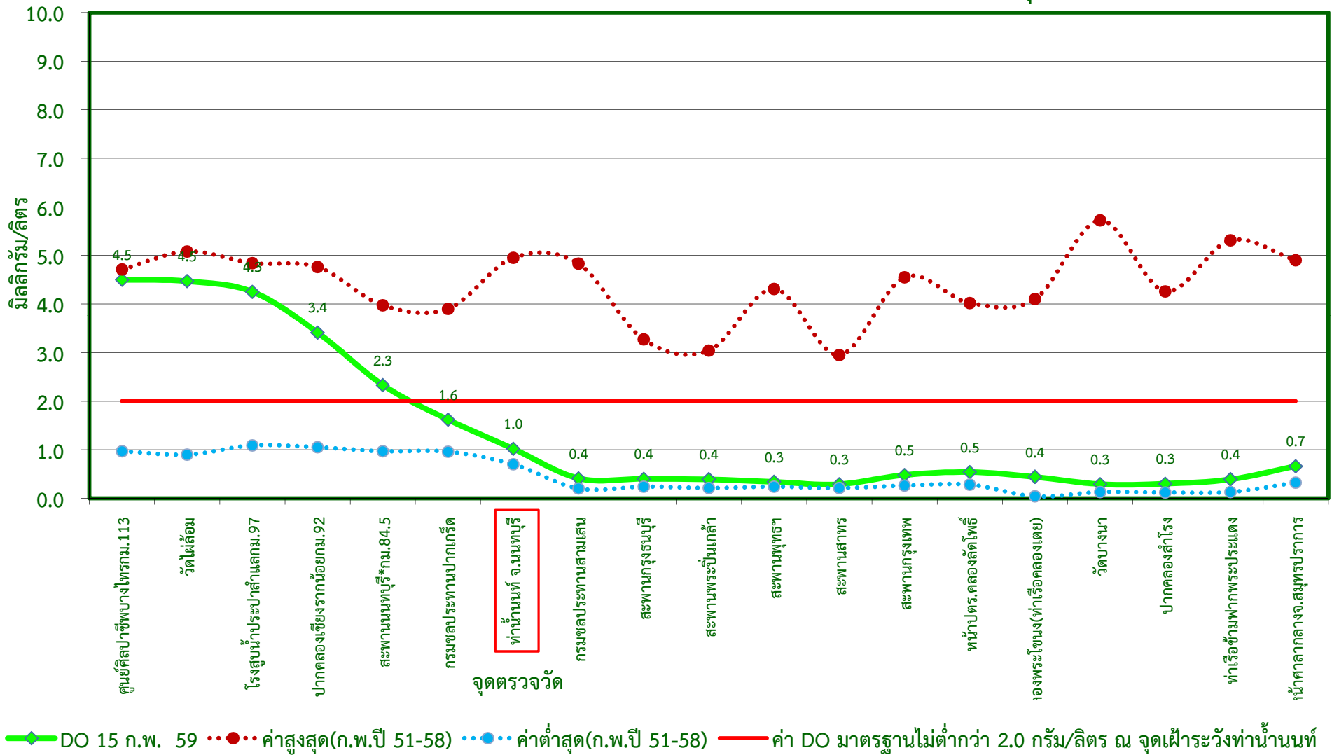
กราฟแสดงค่าออกซิเจนละลายน้ำในแม่น้ำเจ้าพระยาตามพระราชเสาวนีย์ฯ เมื่อวันที่ 15 กุมภาพันธ์ 2559
