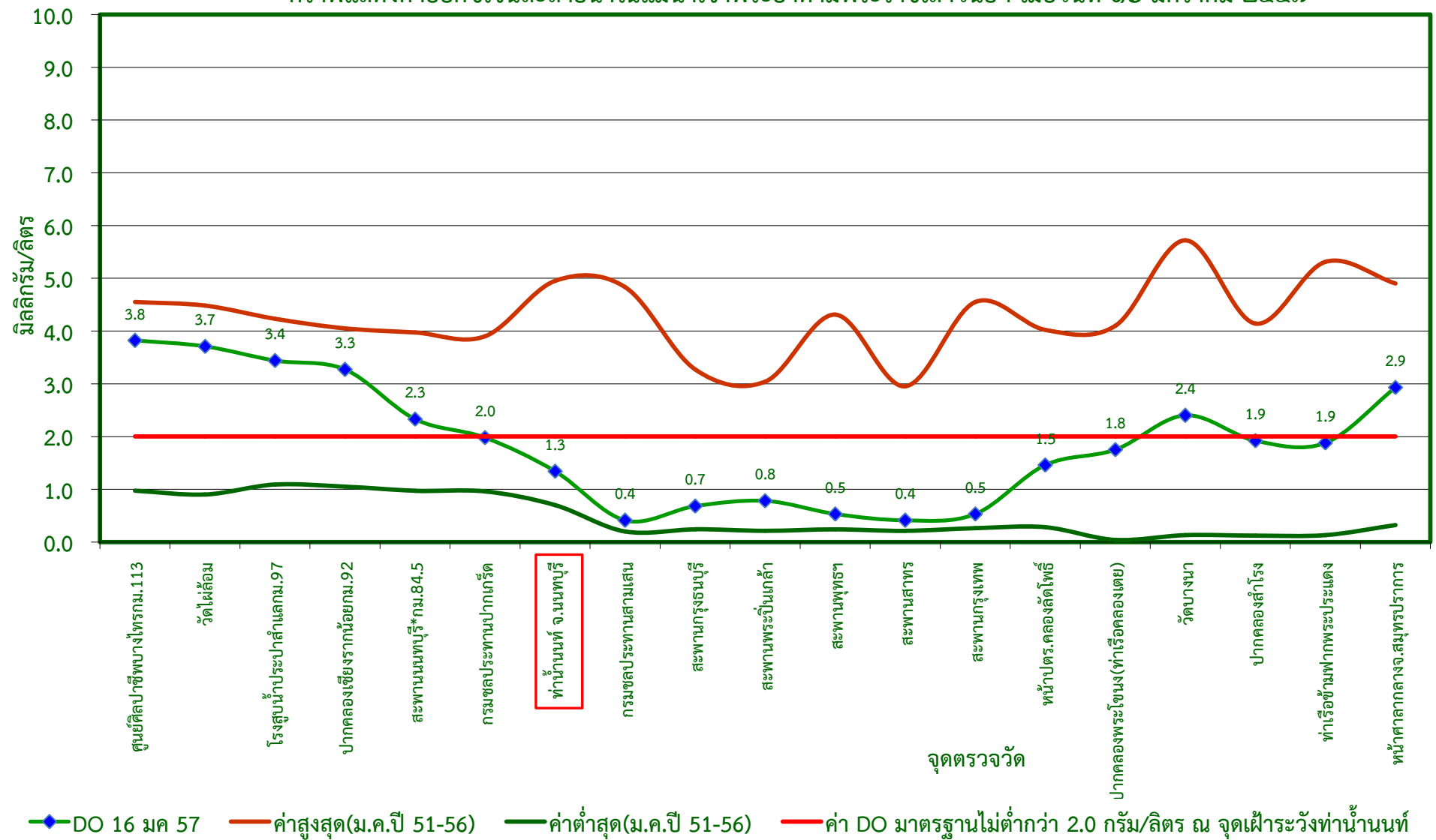
กราฟแสดงค่าออกซิเจนละลายน้ำในแม่น้ำเจ้าพระยาตามพระราชเสาวนีย์ฯ เมื่อวันที่ ๑๖ มกราคม ๒๕๕๗
