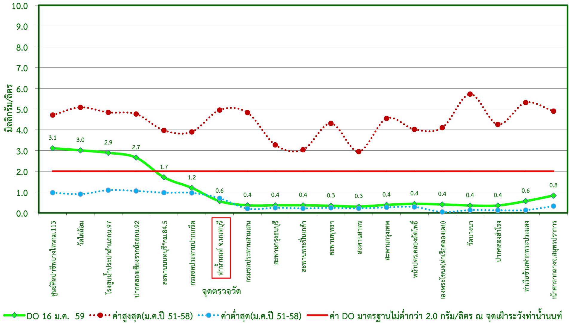
กราฟแสดงค่าออกซิเจนละลายน้ำในแม่น้ำเจ้าพระยาตามพระราชเสาวนีย์ฯ เมื่อวันที่ 16 มกราคม 2559
