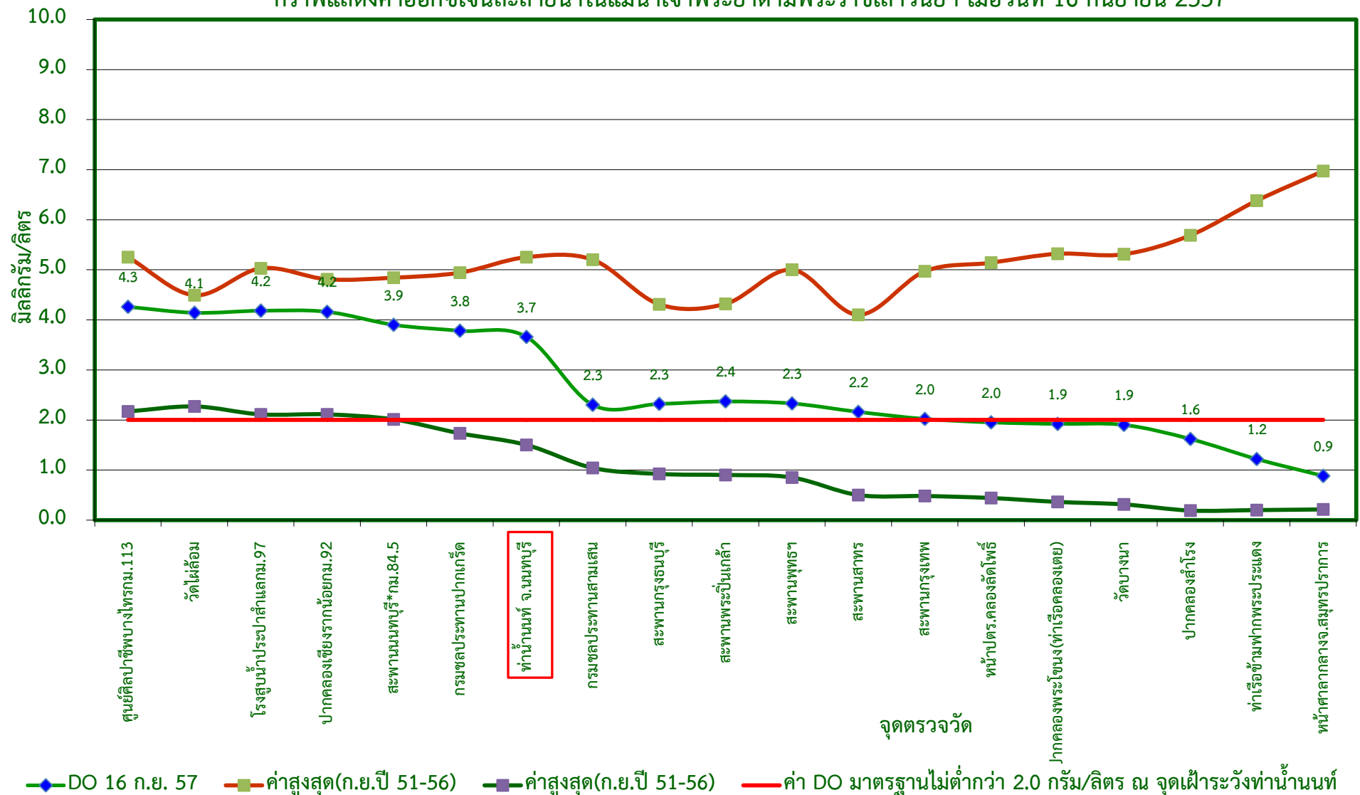
กราฟแสดงค่าออกซิเจนละลายน้ำในแม่น้ำเจ้าพระยาตามพระราชเสาวนีย์ฯ เมื่อวันที่ 16 กันยายน 2557
