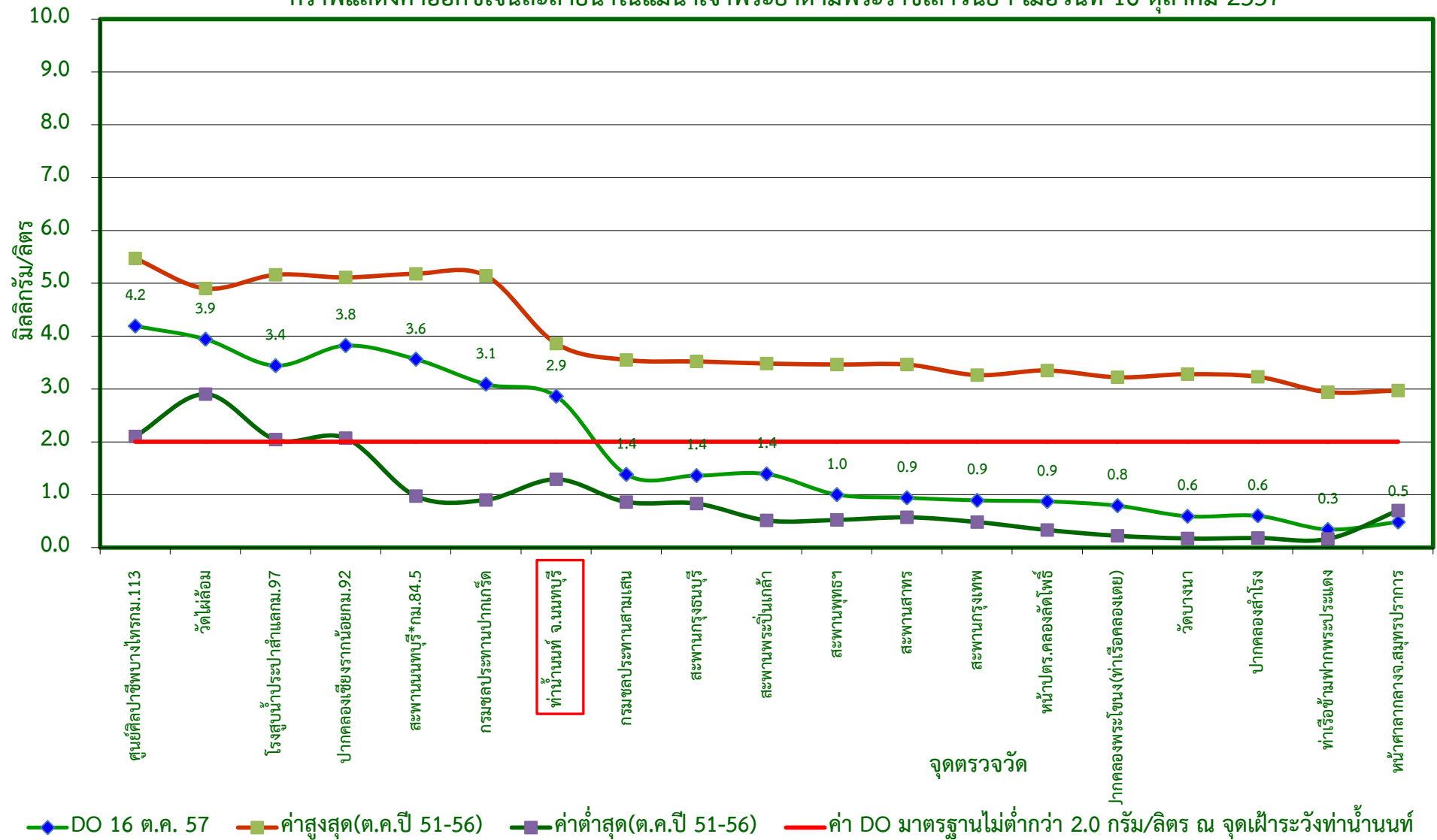
กราฟแสดงค่าออกซิเจนละลายน้ำในแม่น้ำเจ้าพระยาตามพระราชเสาวนีย์ฯ เมื่อวันที่ 16 ตุลาคม 2557
