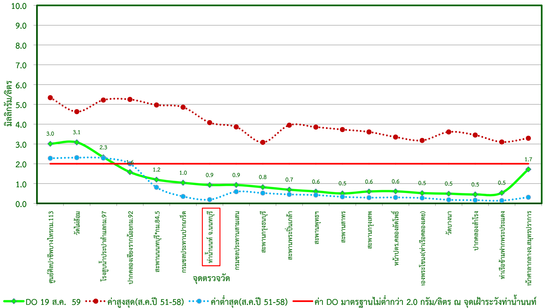
กราฟแสดงค่าออกซิเจนละลายน้ำในแม่น้ำเจ้าพระยาตามพระราชเสาวนีย์ฯ เมื่อวันที่ 19 สิงหาคม 2559
