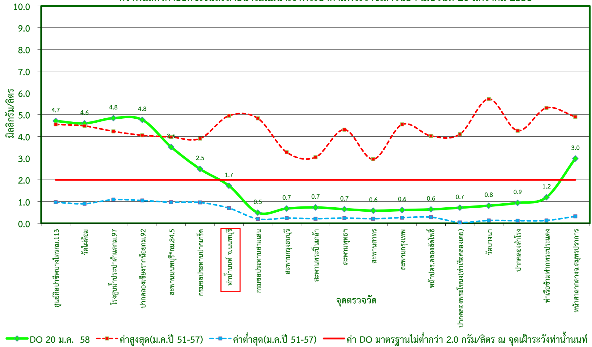
กราฟแสดงค่าออกซิเจนละลายน้ำในแม่น้ำเจ้าพระยาตามพระราชเสาวนีย์ฯ เมื่อวันที่ 20 มกราคม 2558
