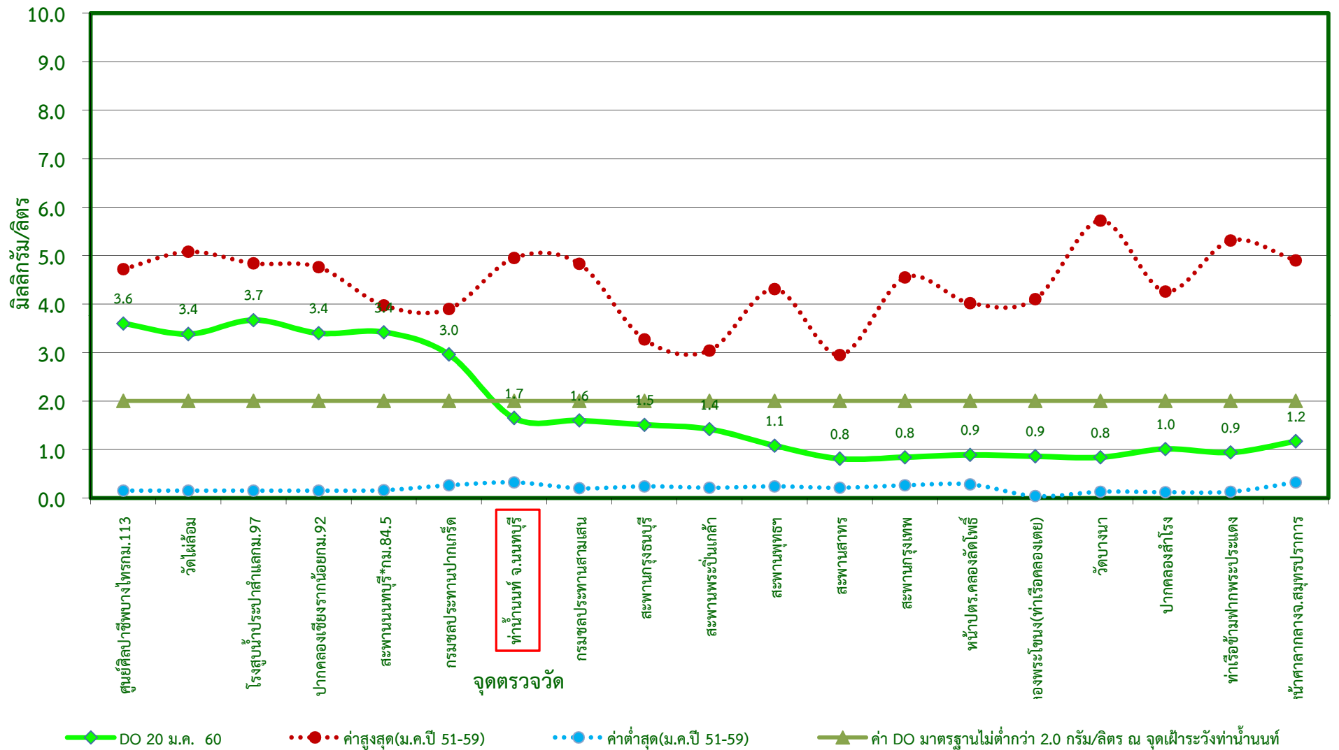
กราฟแสดงค่าออกซิเจนละลายน้ำในแม่น้ำเจ้าพระยาตามพระราชเสาวนีย์ฯ เมื่อวันที่ 20 มกราคม 2560
