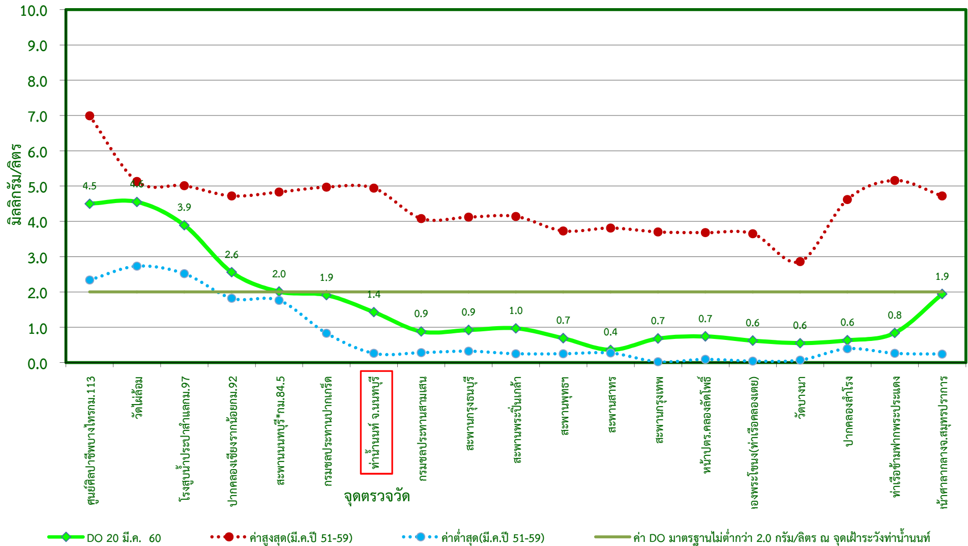
กราฟแสดงค่าออกซิเจนละลายน้ำในแม่น้ำเจ้าพระยาตามพระราชเสาวนีย์ฯ เมื่อวันที่ 20 มีนาคม 2560
