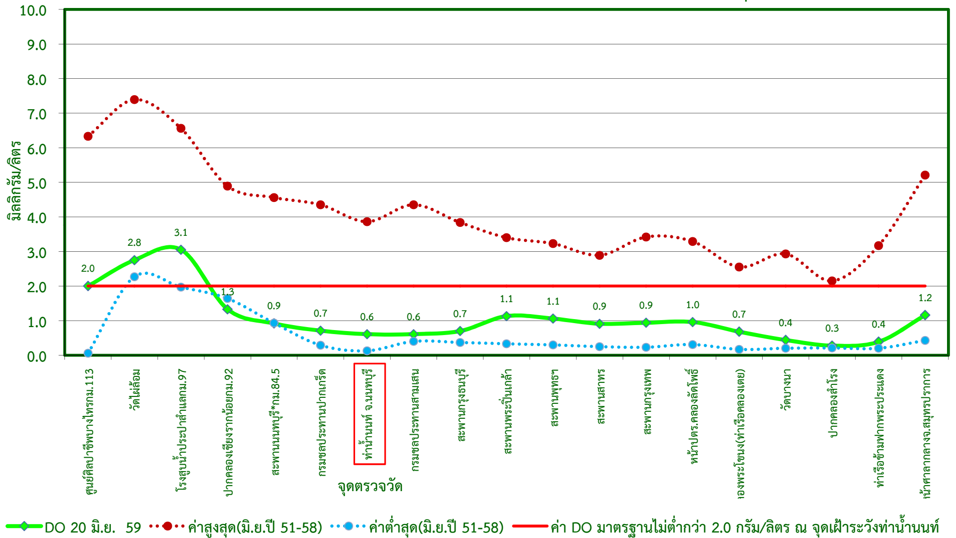
กราฟแสดงค่าออกซิเจนละลายน้ำในแม่น้ำเจ้าพระยาตามพระราชเสาวนีย์ฯ เมื่อวันที่ 20 มิถุนายน 2559
