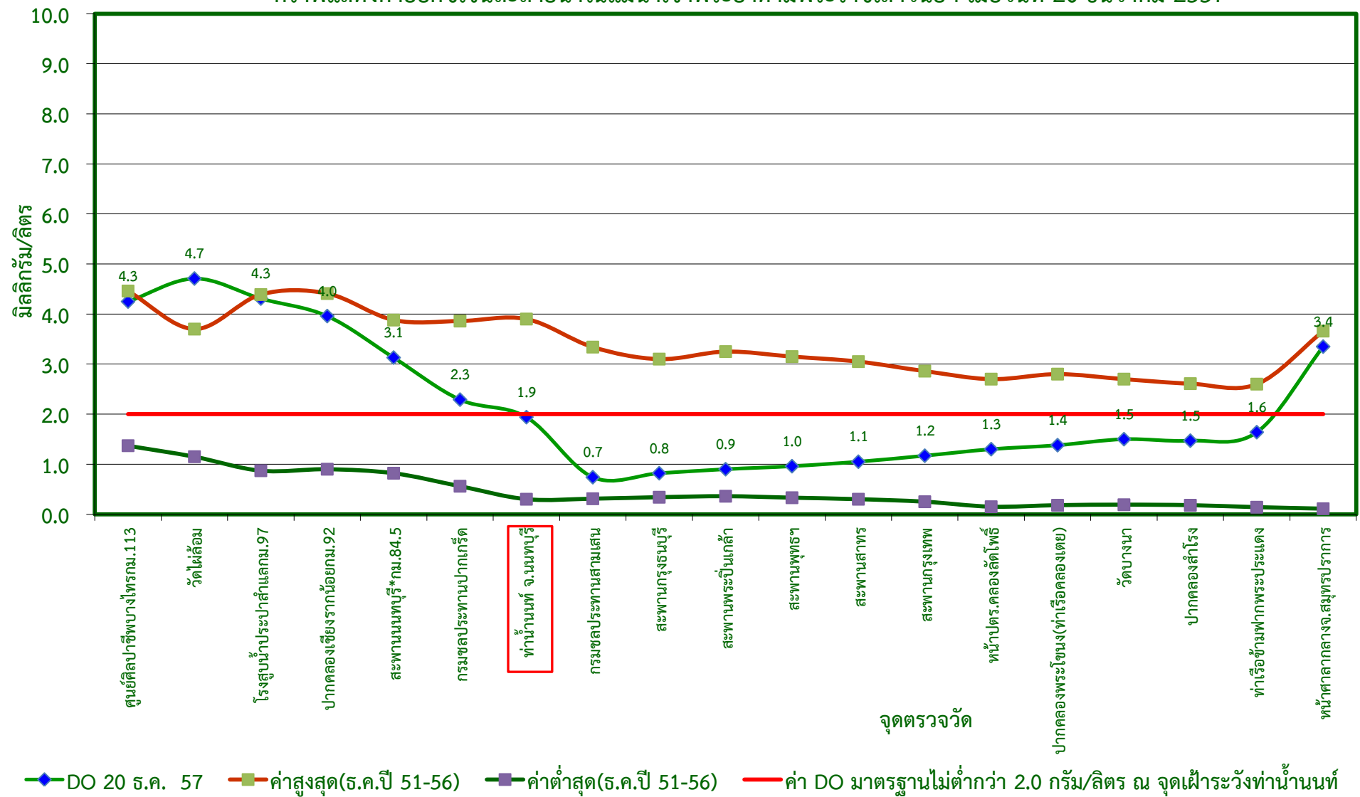
กราฟแสดงค่าออกซิเจนละลายน้ำในแม่น้ำเจ้าพระยาตามพระราชเสาวนีย์ฯ เมื่อวันที่ 20 ธันวาคม 2557
