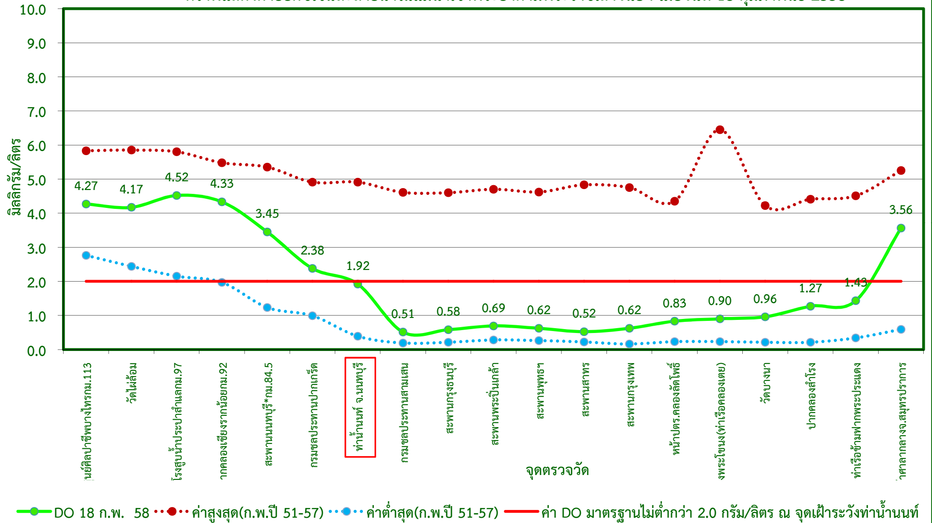
กราฟแสดงค่าออกซิเจนละลายน้ำในแม่น้ำเจ้าพระยาตามพระราชเสาวนีย์ฯ เมื่อวันที่ 18 กุมภาพันธ์ 2558
