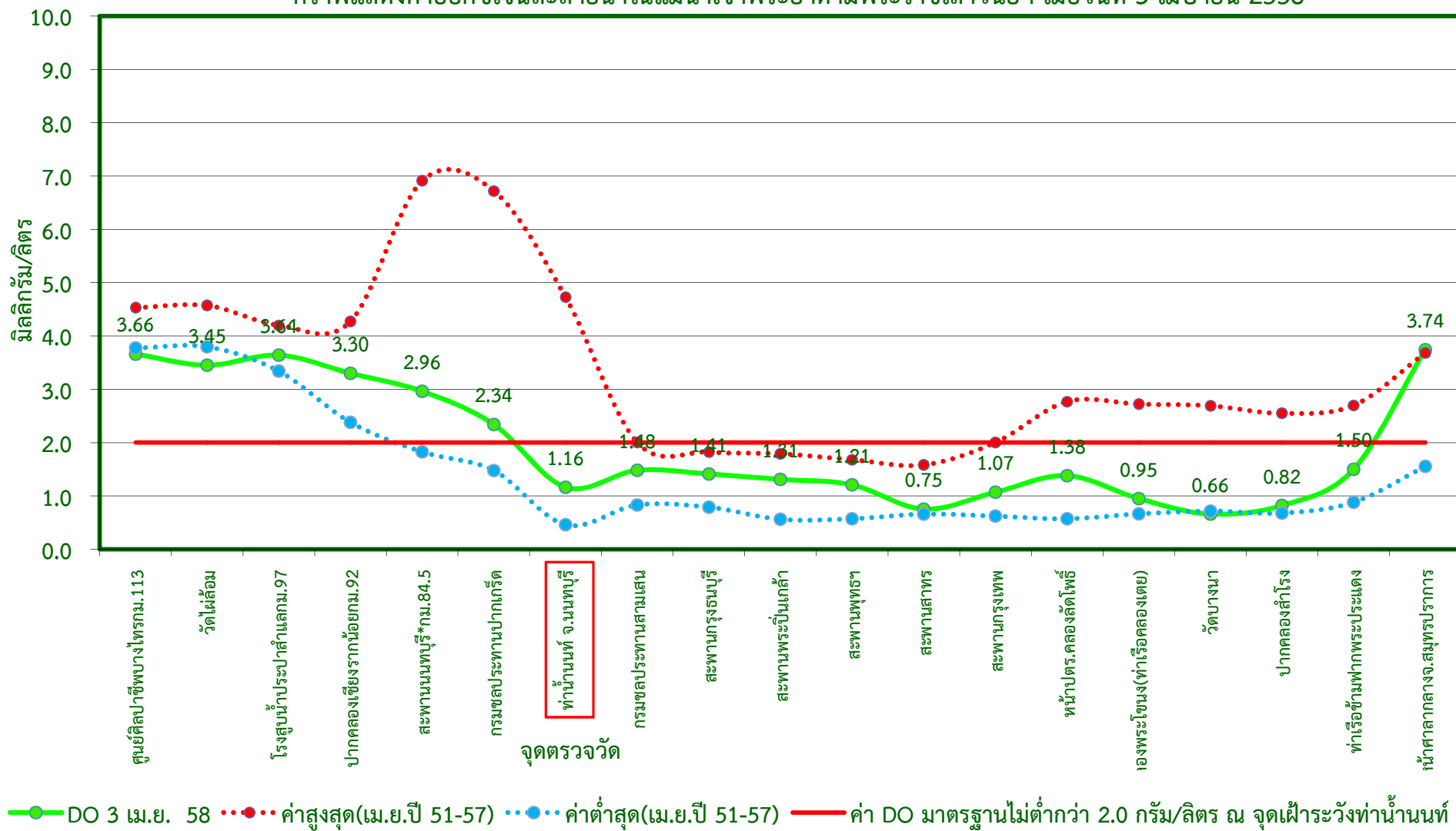
กราฟแสดงค่าออกซิเจนละลายน้ำในแม่น้ำเจ้าพระยาตามพระราชเสาวนีย์ฯ เมื่อวันที่ 3 เมษายน 2558
