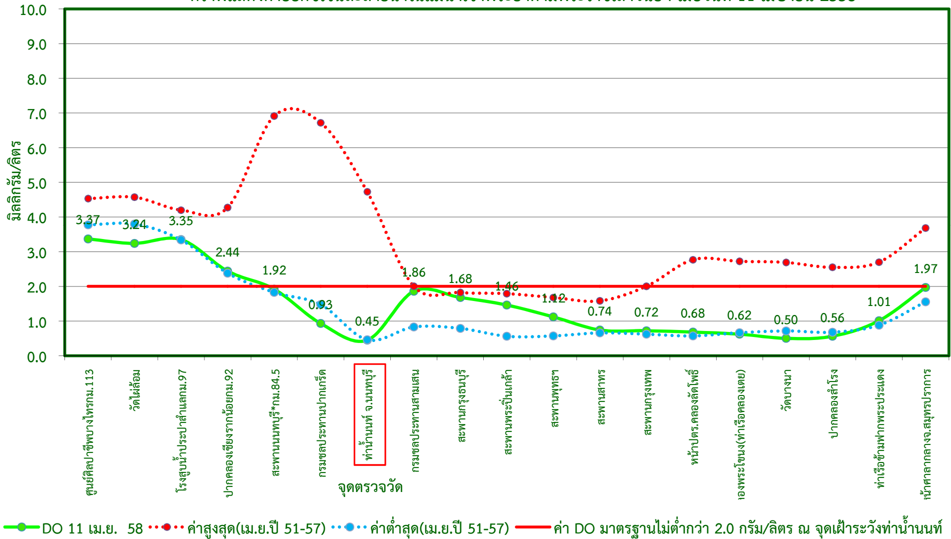
กราฟแสดงค่าออกซิเจนละลายน้ำในแม่น้ำเจ้าพระยาตามพระราชเสาวนีย์ฯ เมื่อวันที่ 11 เมษายน 2558
