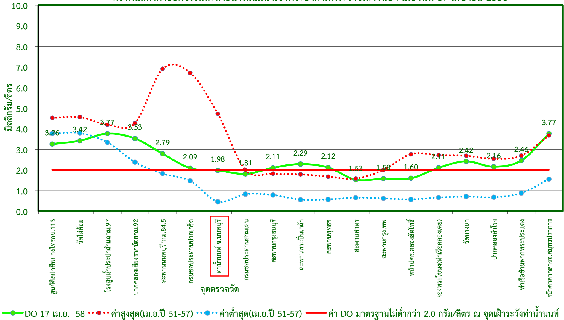
กราฟแสดงค่าออกซิเจนละลายน้ำในแม่น้ำเจ้าพระยาตามพระราชเสาวนีย์ฯ เมื่อวันที่ 17 เมษายน 2558
