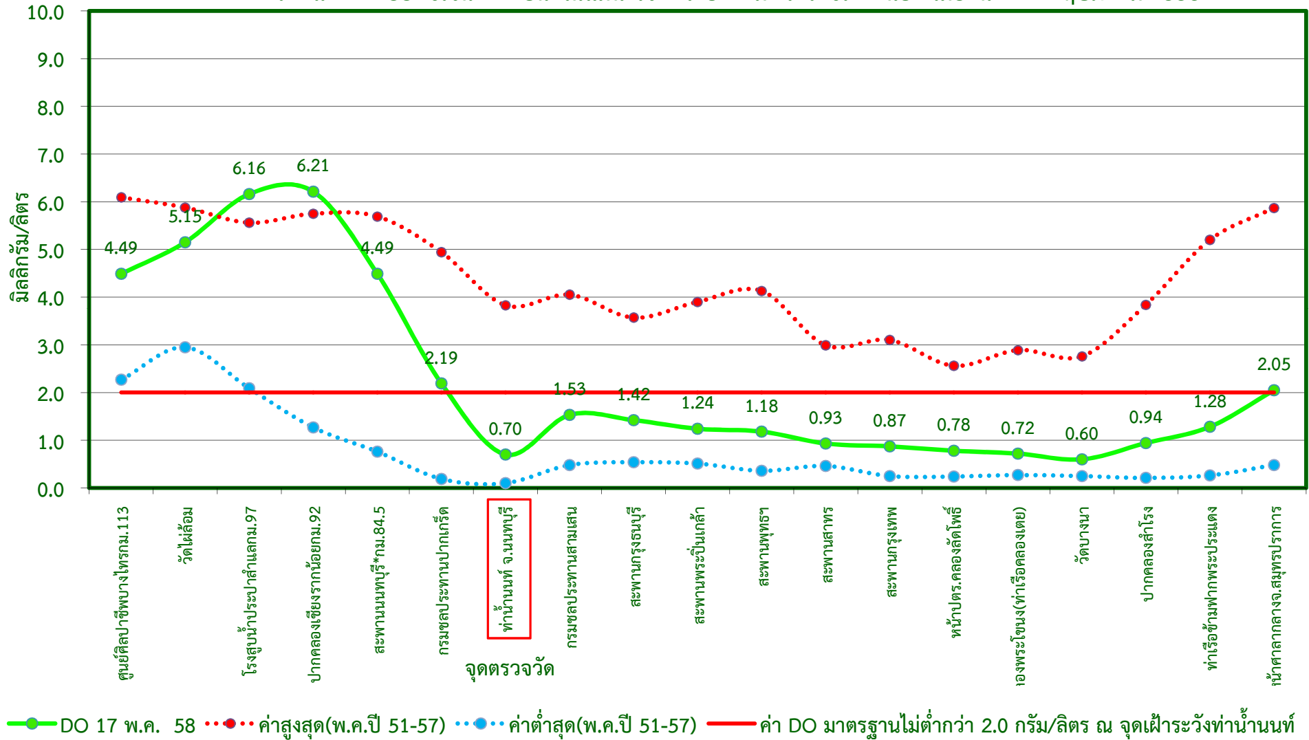
กราฟแสดงค่าออกซิเจนละลายน้ำในแม่น้ำเจ้าพระยาตามพระราชเสาวนีย์ฯ เมื่อวันที่ 17 พฤษภาคม 2558
