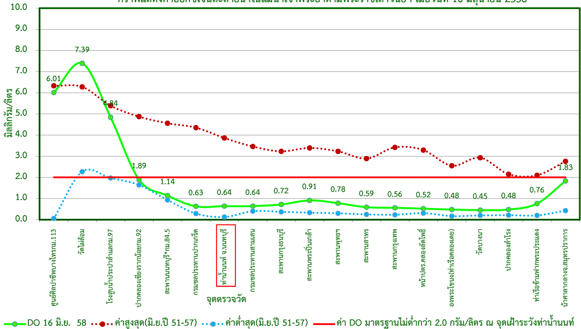
กราฟแสดงค่าออกซิเจนละลายน้ำในแม่น้ำเจ้าพระยาตามพระราชเสาวนีย์ฯ เมื่อวันที่ 16 มิถุนายน 2558
