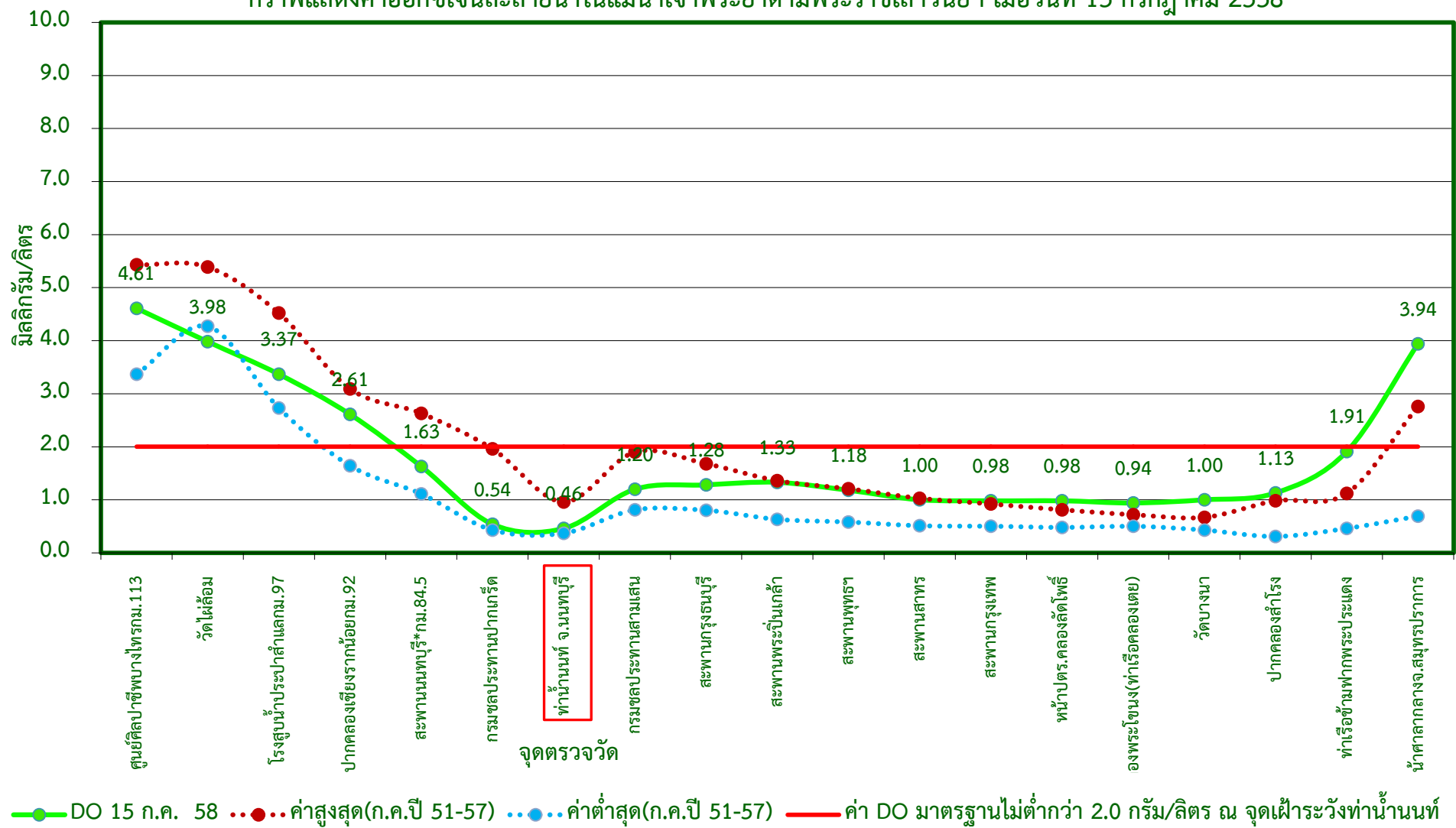
กราฟแสดงค่าออกซิเจนละลายน้ำในแม่น้ำเจ้าพระยาตามพระราชเสาวนีย์ฯ เมื่อวันที่ 15 กรกฎาคม 2558
