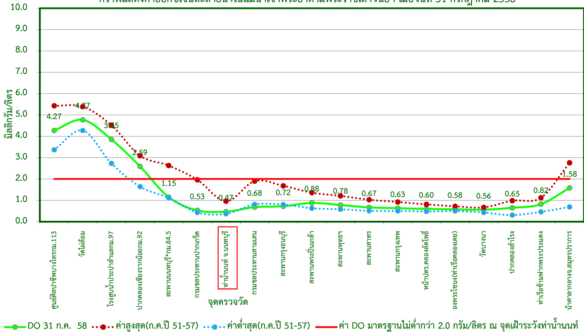
กราฟแสดงค่าออกซิเจนละลายน้ำในแม่น้ำเจ้าพระยาตามพระราชเสาวนีย์ฯ เมื่อวันที่ 31 กรกฎาคม 2558
