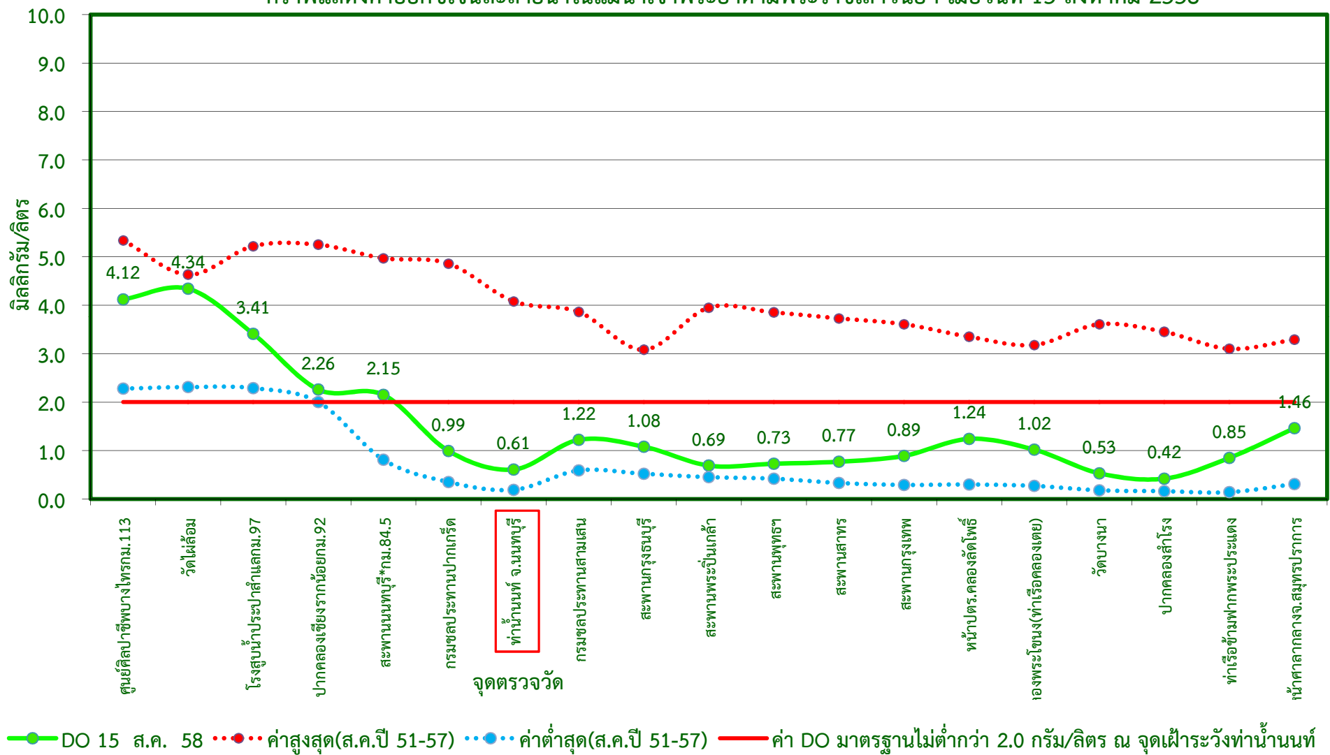
กราฟแสดงค่าออกซิเจนละลายน้ำในแม่น้ำเจ้าพระยาตามพระราชเสาวนีย์ฯ เมื่อวันที่ 15 สิงหาคม 2558
