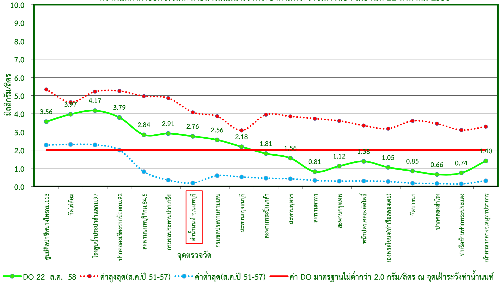
กราฟแสดงค่าออกซิเจนละลายน้ำในแม่น้ำเจ้าพระยาตามพระราชเสาวนีย์ฯ เมื่อวันที่ 22 สิงหาคม 2558
