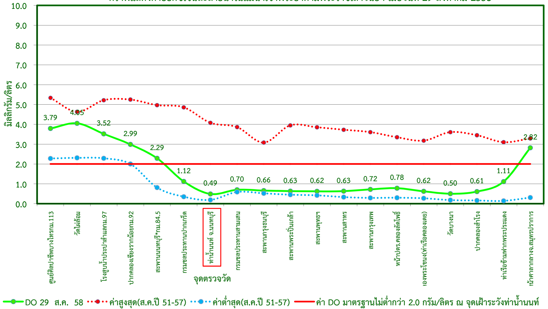
กราฟแสดงค่าออกซิเจนละลายน้ำในแม่น้ำเจ้าพระยาตามพระราชเสาวนีย์ฯ เมื่อวันที่ 29 สิงหาคม 2558
