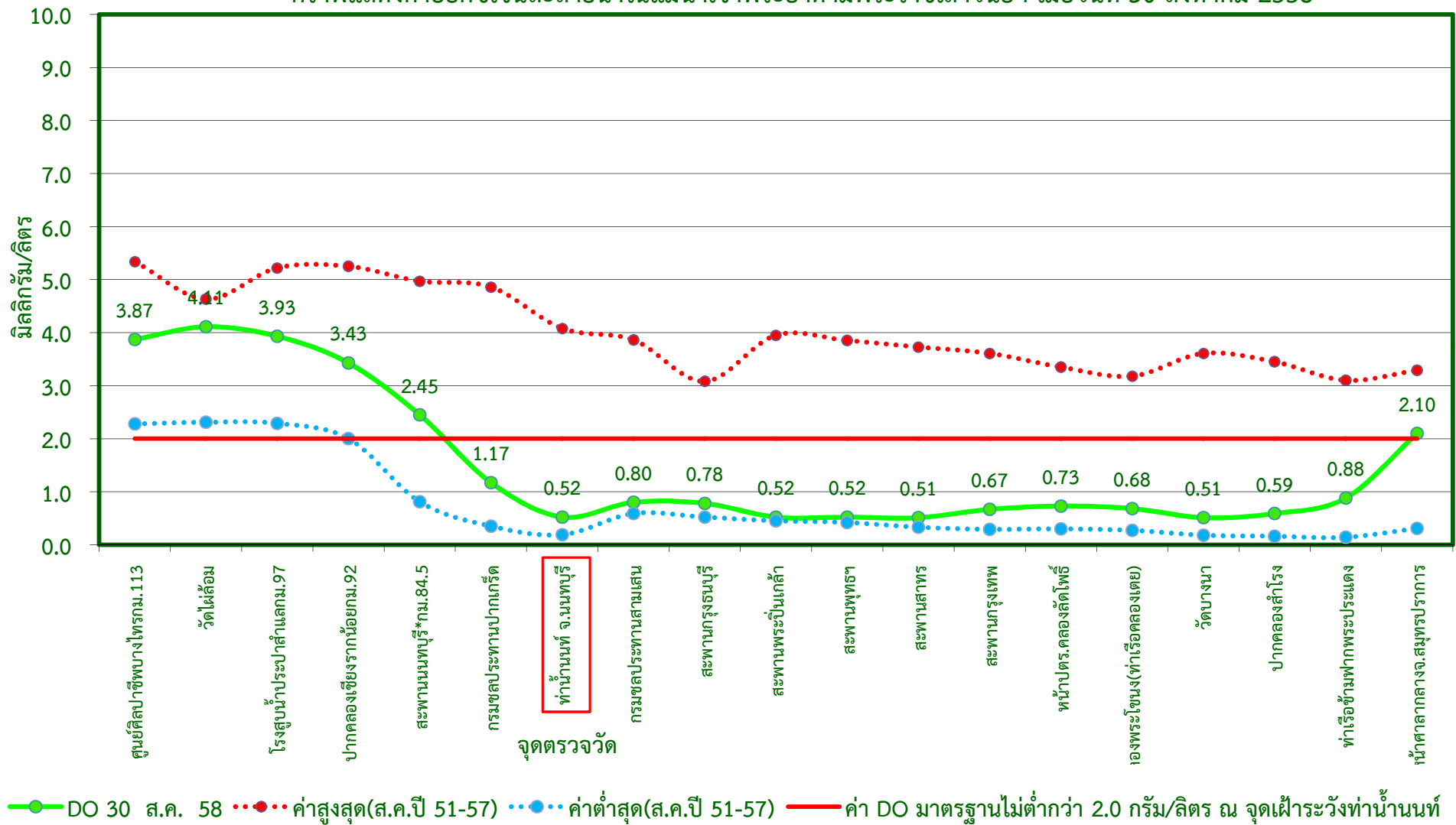
กราฟแสดงค่าออกซิเจนละลายน้ำในแม่น้ำเจ้าพระยาตามพระราชเสาวนีย์ฯ เมื่อวันที่ 30 สิงหาคม 2558
