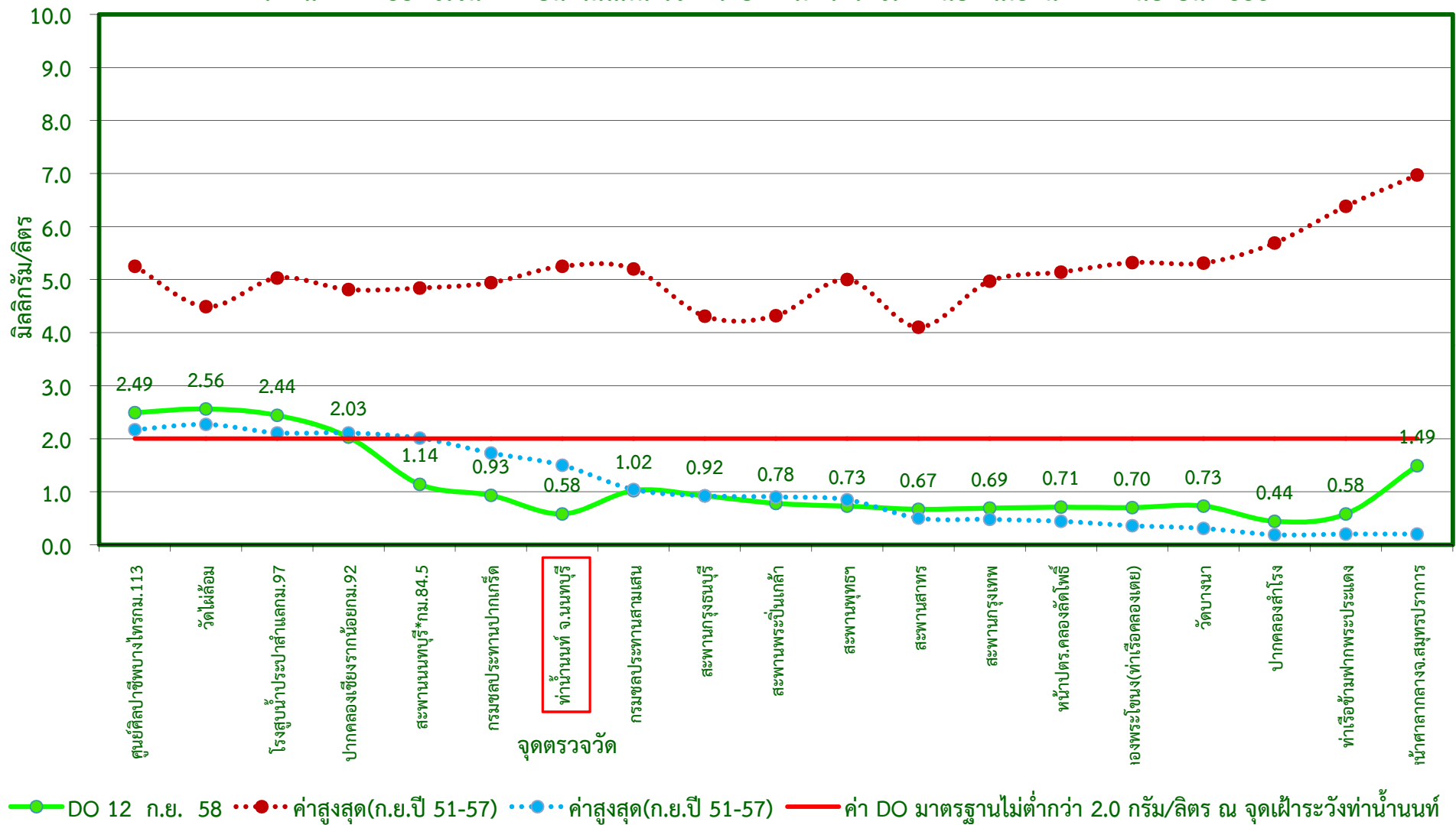
กราฟแสดงค่าออกซิเจนละลายน้ำในแม่น้ำเจ้าพระยาตามพระราชเสาวนีย์ฯ เมื่อวันที่ 12 กันยายน 2558
