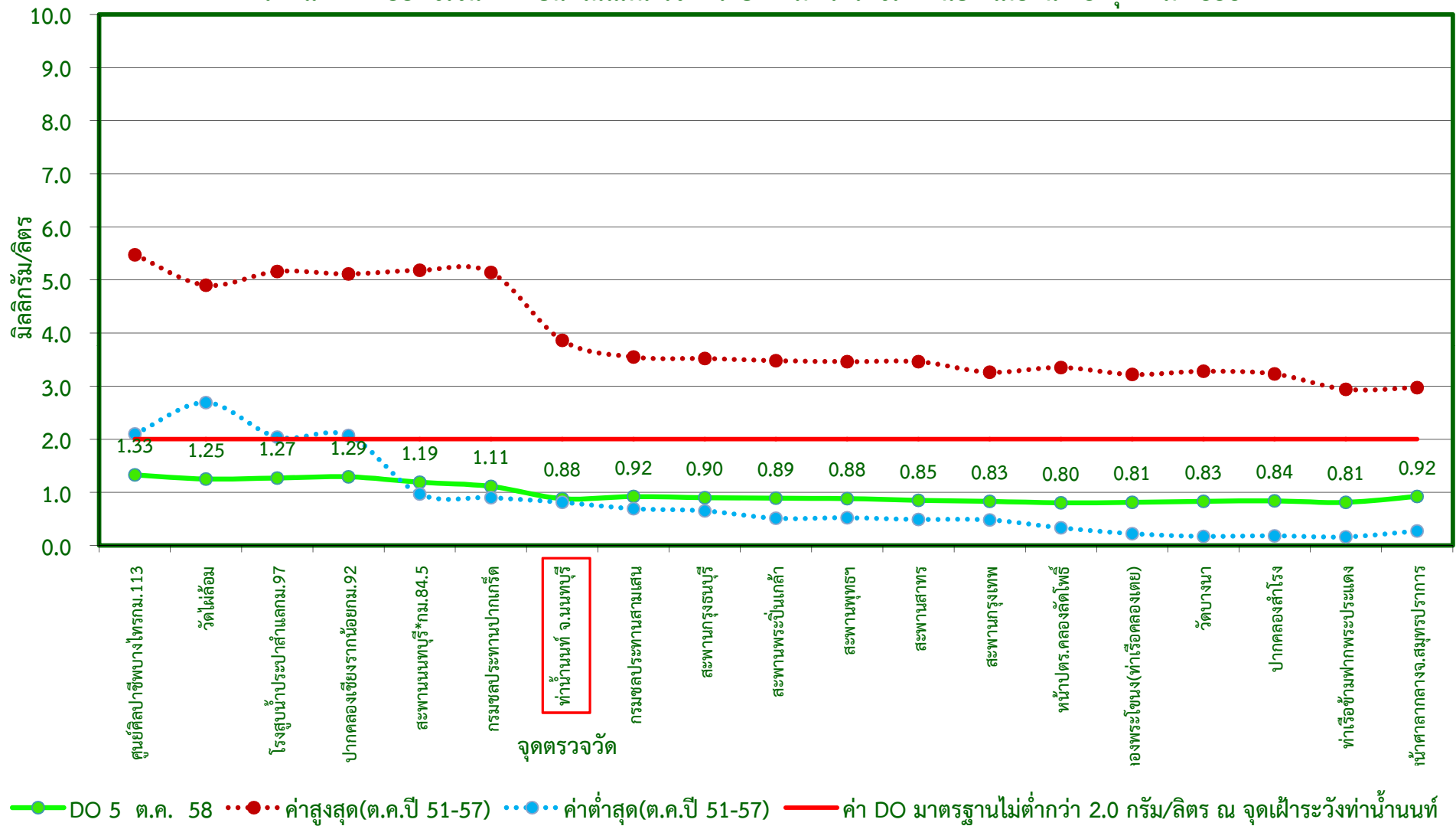
กราฟแสดงค่าออกซิเจนละลายน้ำในแม่น้ำเจ้าพระยาตามพระราชเสาวนีย์ฯ เมื่อวันที่ 5 ตุลาคม 2558
