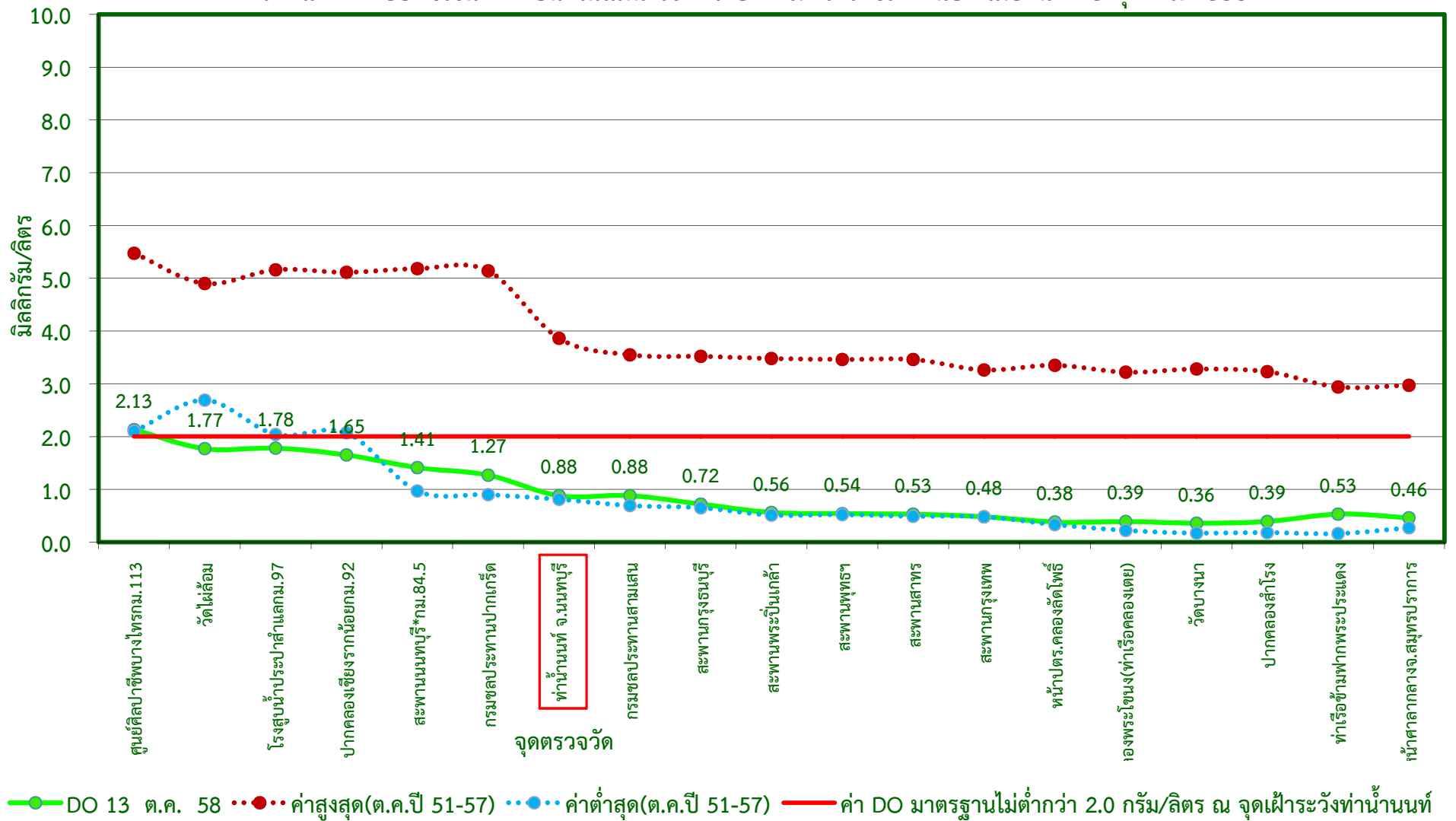
กราฟแสดงค่าออกซิเจนละลายน้ำในแม่น้ำเจ้าพระยาตามพระราชเสาวนีย์ฯ เมื่อวันที่ 13 ตุลาคม 2558
