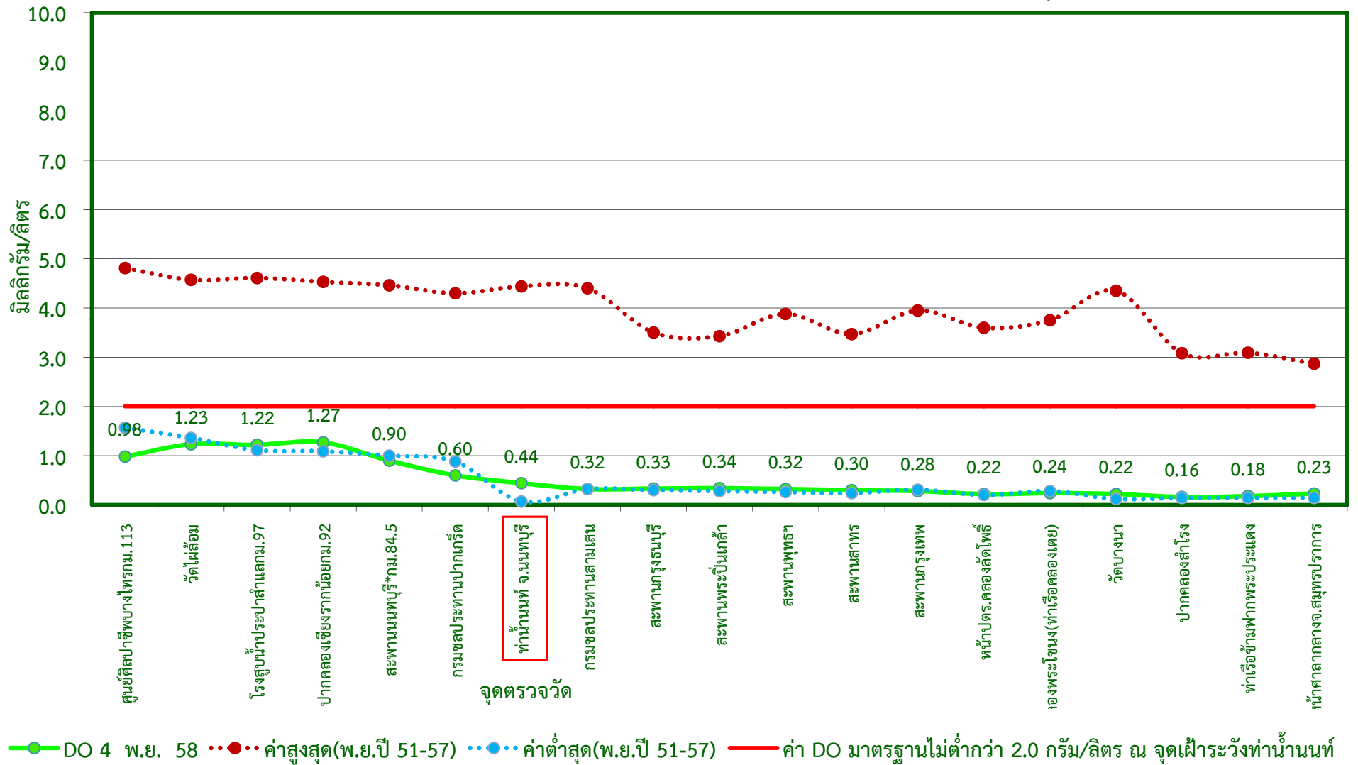
กราฟแสดงค่าออกซิเจนละลายน้ำในแม่น้ำเจ้าพระยาตามพระราชเสาวนีย์ฯ เมื่อวันที่ 4 พฤศจิกายน 2558
