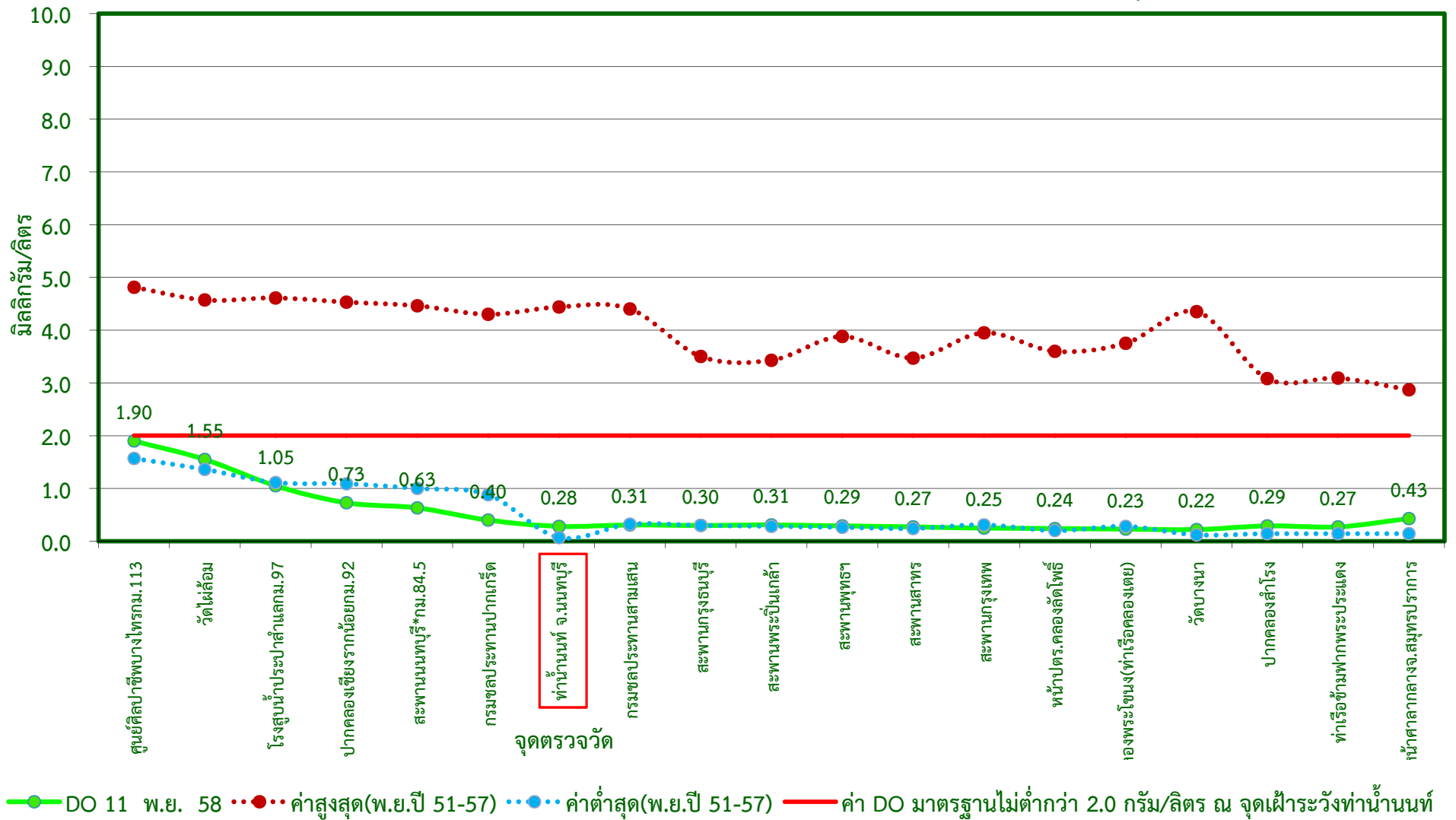
กราฟแสดงค่าออกซิเจนละลายน้ำในแม่น้ำเจ้าพระยาตามพระราชเสาวนีย์ฯ เมื่อวันที่ 11 พฤศจิกายน 2558
