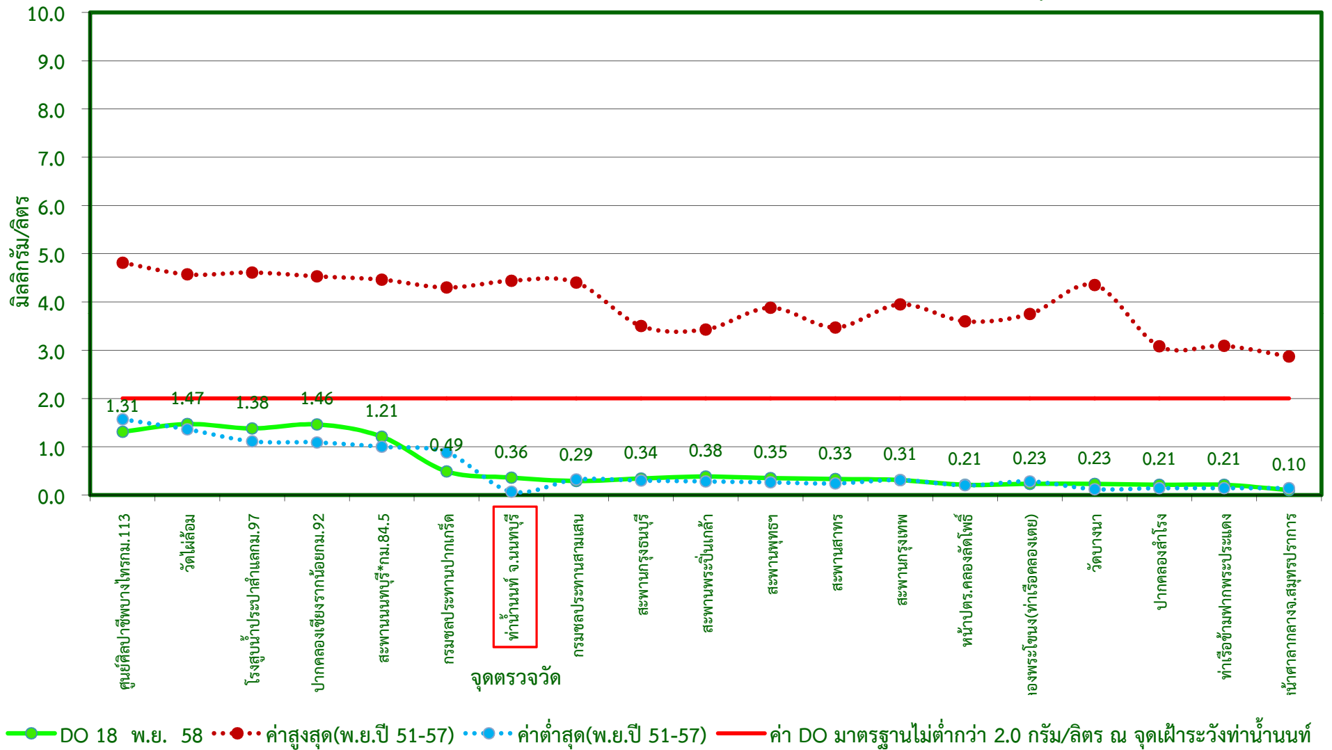
กราฟแสดงค่าออกซิเจนละลายน้ำในแม่น้ำเจ้าพระยาตามพระราชเสาวนีย์ฯ เมื่อวันที่ 18 พฤศจิกายน 2558
