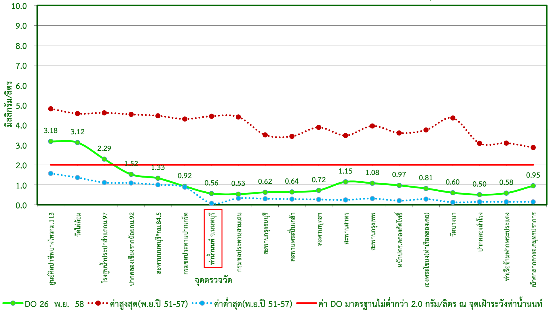
กราฟแสดงค่าออกซิเจนละลายน้ำในแม่น้ำเจ้าพระยาตามพระราชเสาวนีย์ฯ เมื่อวันที่ 26 พฤศจิกายน 2558
