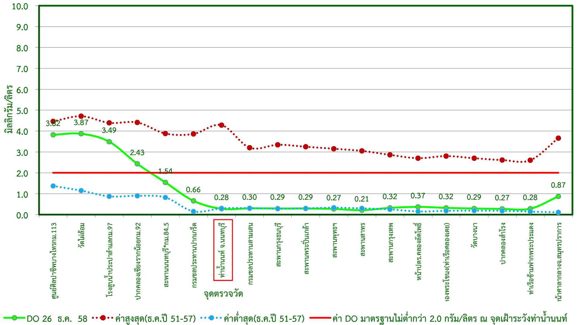
กราฟแสดงค่าออกซิเจนละลายน้ำในแม่น้ำเจ้าพระยาตามพระราชเสาวนีย์ฯ เมื่อวันที่ 26 ธันวาคม 2558
