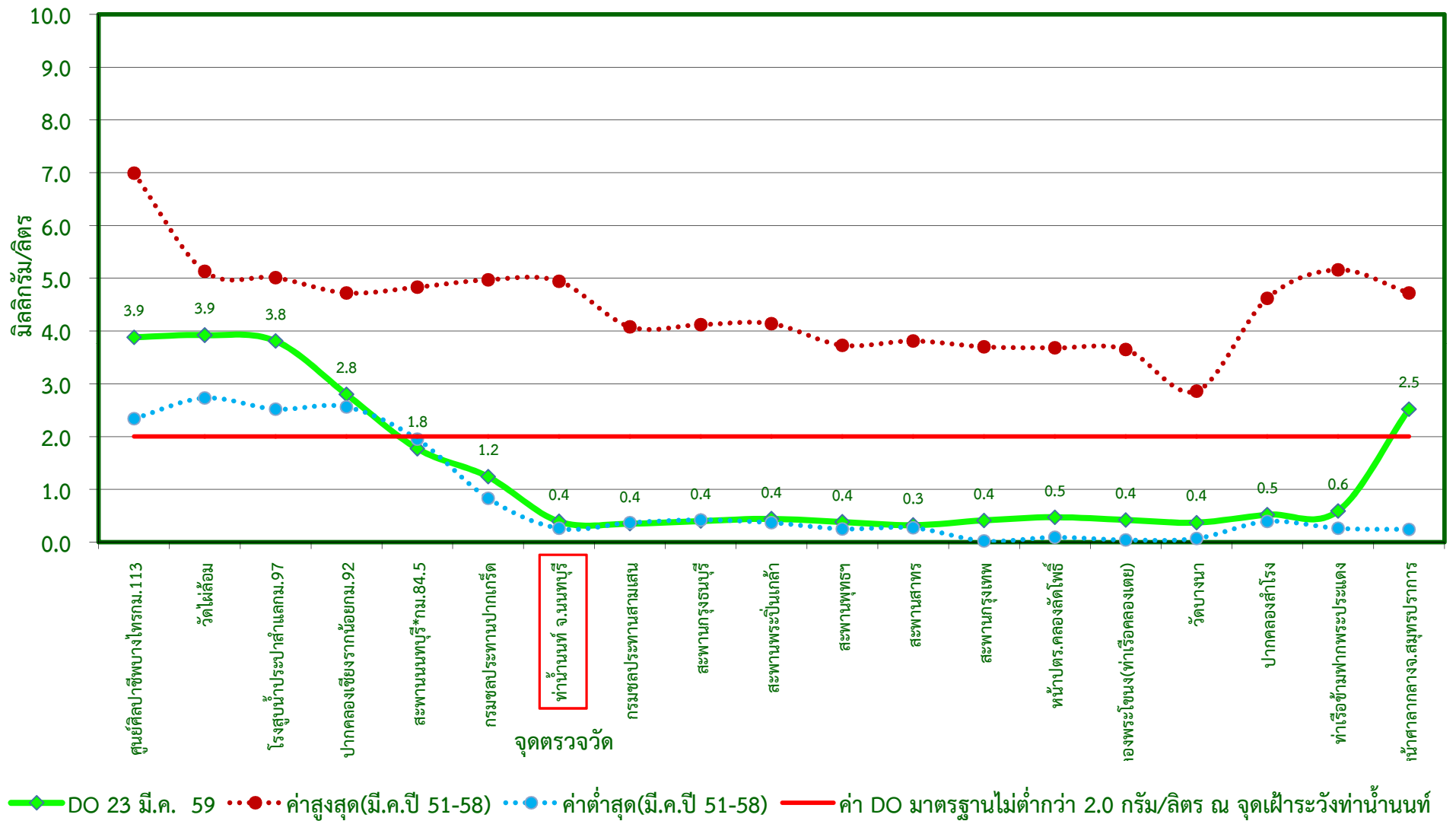
กราฟแสดงค่าออกซิเจนละลายน้ำในแม่น้ำเจ้าพระยาตามพระราชเสาวนีย์ฯ เมื่อวันที่ 23 มีนาคม 2559
