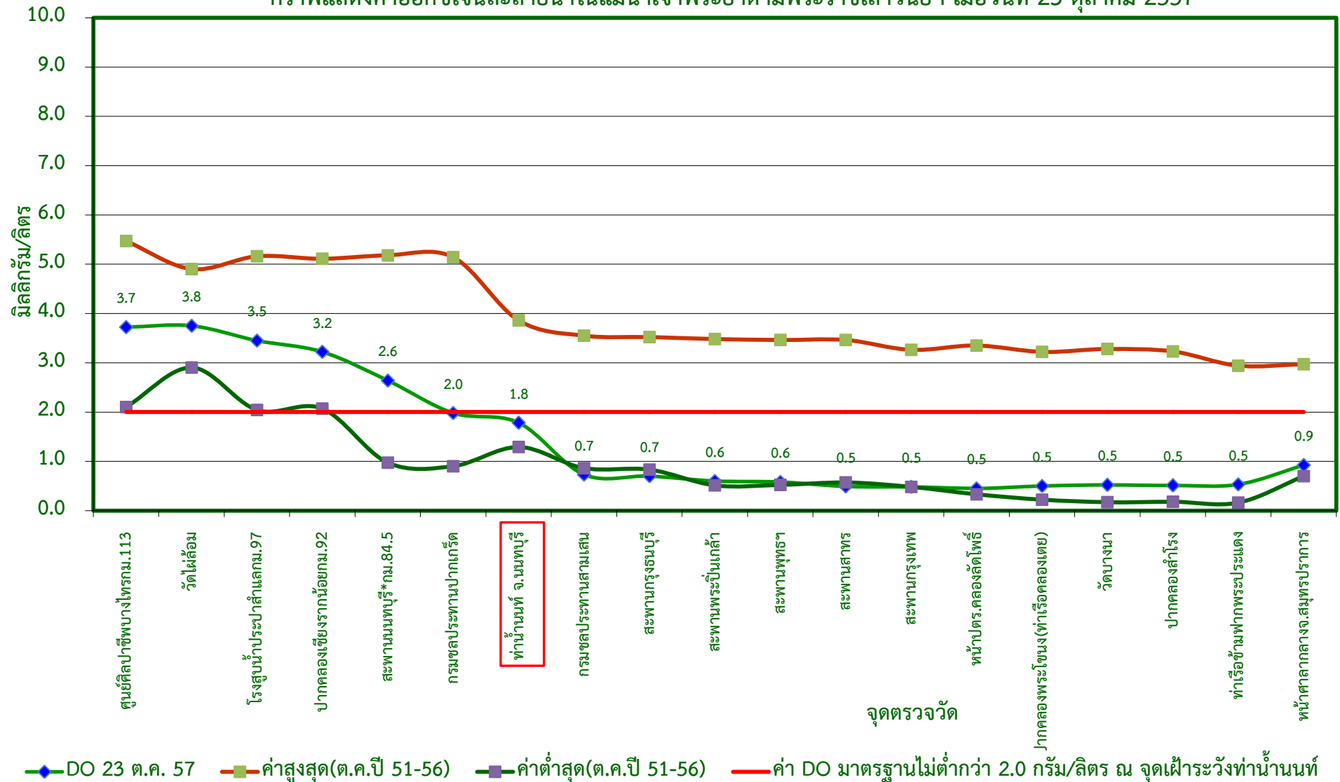
กราฟแสดงค่าออกซิเจนละลายน้ำในแม่น้ำเจ้าพระยาตามพระราชเสาวนีย์ฯ เมื่อวันที่ 23 ตุลาคม 2557
