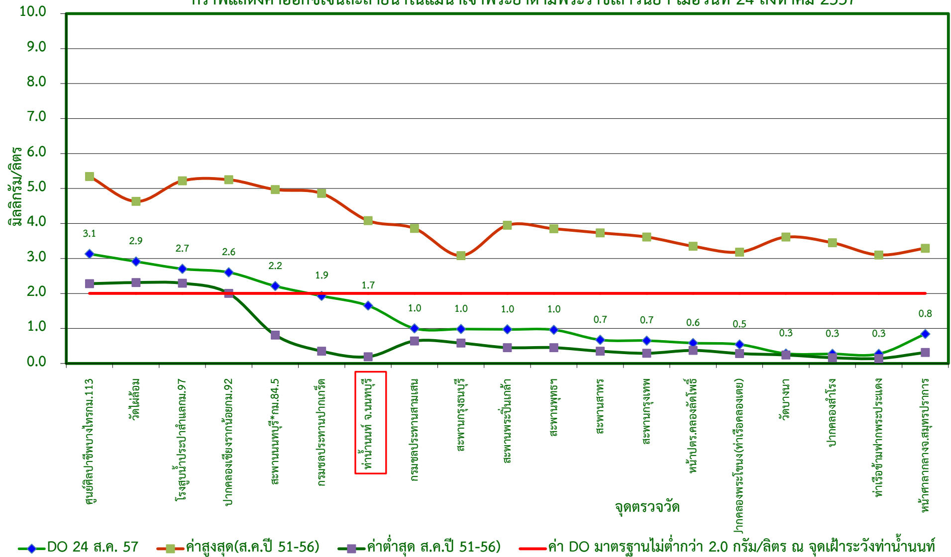
กราฟแสดงค่าออกซิเจนละลายน้ำในแม่น้ำเจ้าพระยาตามพระราชเสาวนีย์ฯ เมื่อวันที่ 24 สิงหาคม 2557
