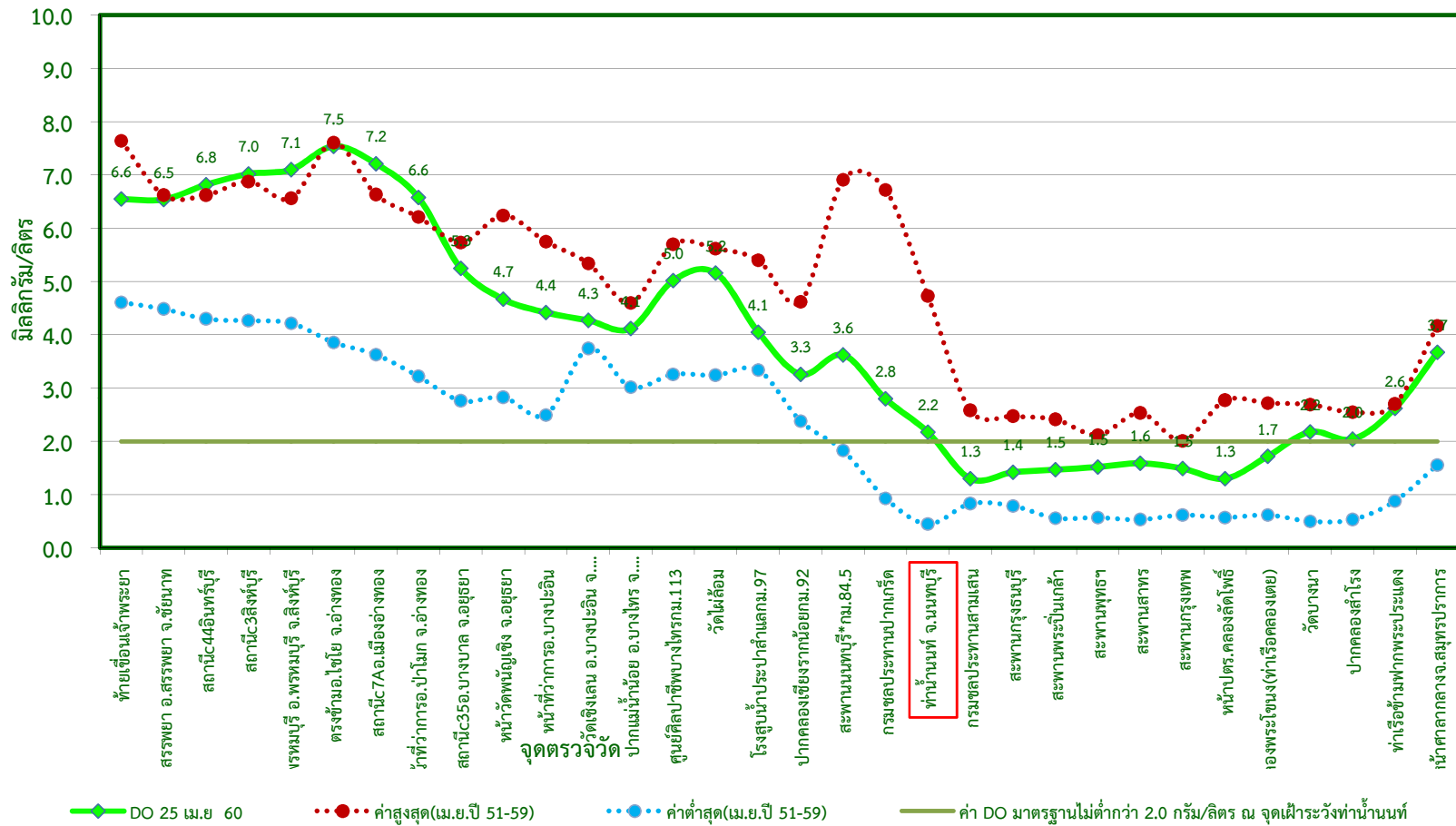
กราฟแสดงค่าออกซิเจนละลายน้ำในแม่น้ำเจ้าพระยาตามพระราชเสาวนีย์ฯ เมื่อวันที่ 25 เมษายน 2560
