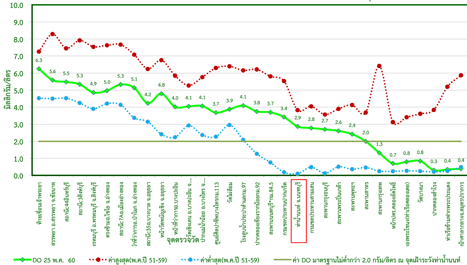
กราฟแสดงค่าออกซิเจนละลายน้ำในแม่น้ำเจ้าพระยาตามพระราชเสาวนีย์ฯ เมื่อวันที่ 25 พฤษภาคม 2560
