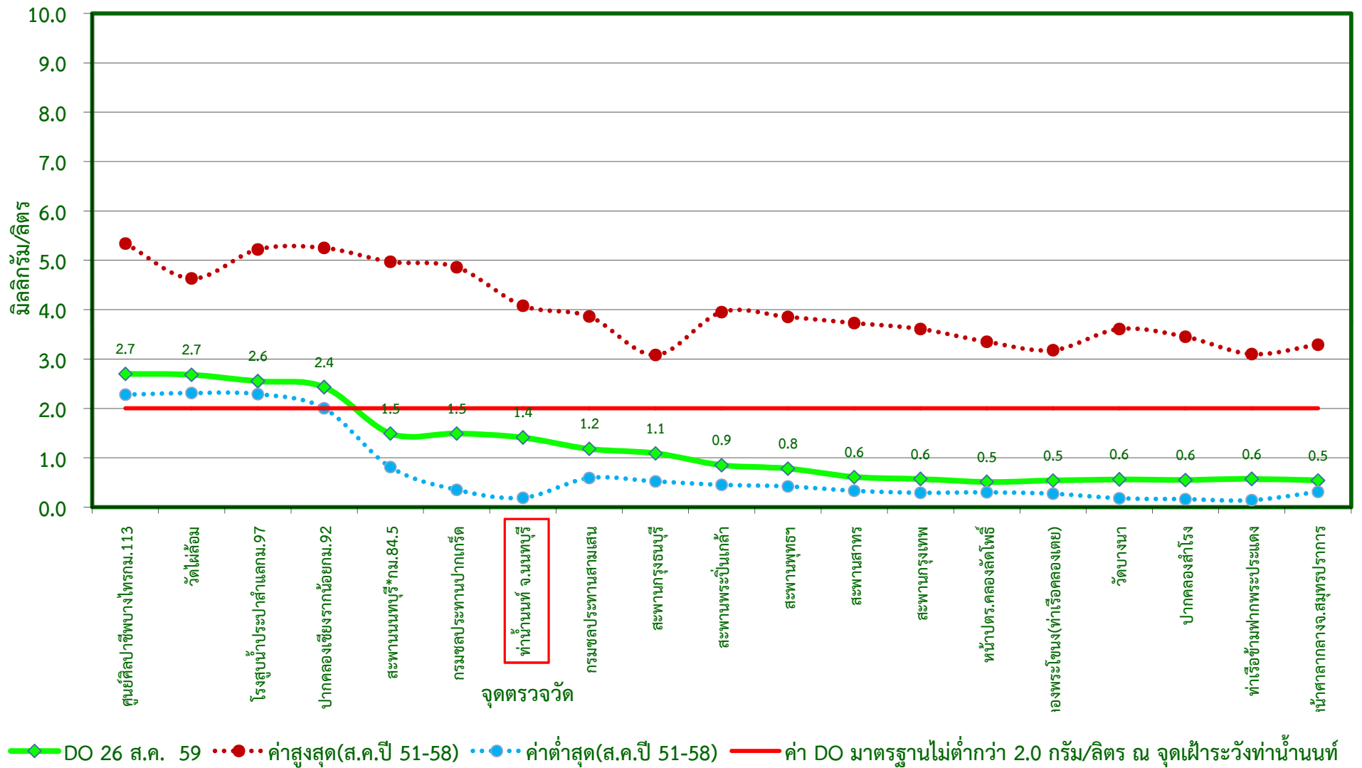
กราฟแสดงค่าออกซิเจนละลายน้ำในแม่น้ำเจ้าพระยาตามพระราชเสาวนีย์ฯ เมื่อวันที่ 26 สิงหาคม 2559
