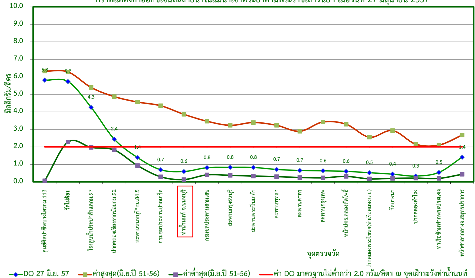
กราฟแสดงค่าออกซิเจนละลายน้ำในแม่น้ำเจ้าพระยาตามพระราชเสาวนีย์ฯ เมื่อวันที่ 27 มิถุนายน 2557
