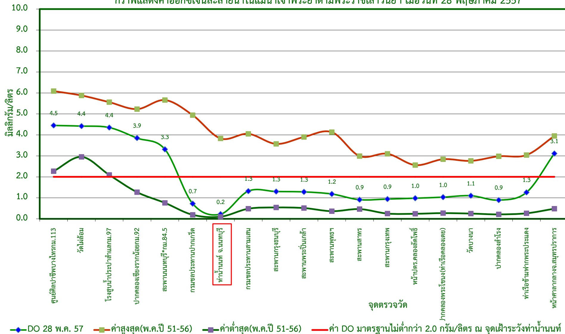
กราฟแสดงค่าออกซิเจนละลายน้ำในแม่น้ำเจ้าพระยาตามพระราชเสาวนีย์ฯ เมื่อวันที่ 28 พฤษภาคม 2557
