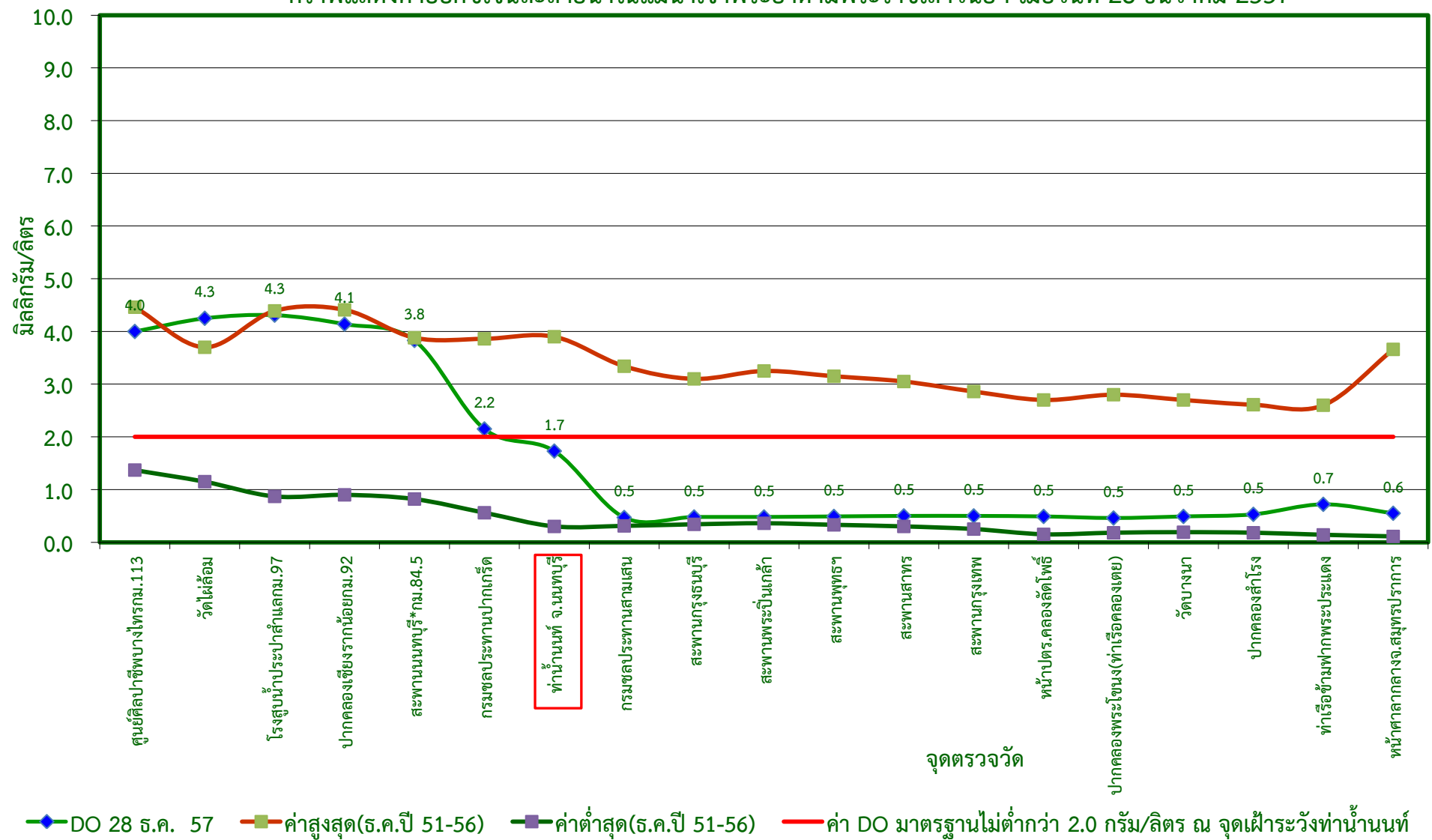
กราฟแสดงค่าออกซิเจนละลายน้ำในแม่น้ำเจ้าพระยาตามพระราชเสาวนีย์ฯ เมื่อวันที่ 28 ธันวาคม 2557
