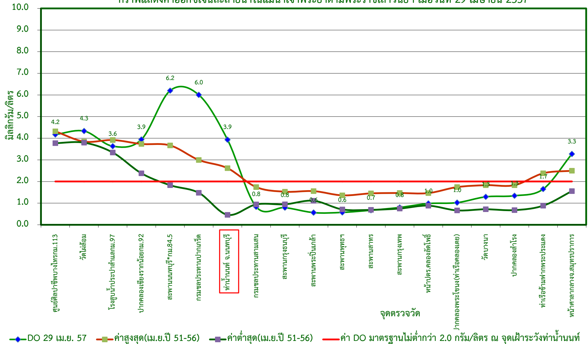
กราฟแสดงค่าออกซิเจนละลายน้ำในแม่น้ำเจ้าพระยาตามพระราชเสาวนีย์ฯ เมื่อวันที่ 29 เมษายน 2557
