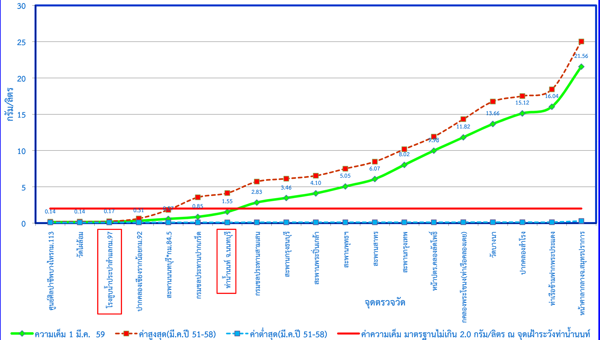
กราฟแสดงค่าความเค็มในแม่น้ำเจ้าพระยาตามพระราชเสาวนีย์ฯ เมื่อวันที่ 1 มีนาคม 2559
