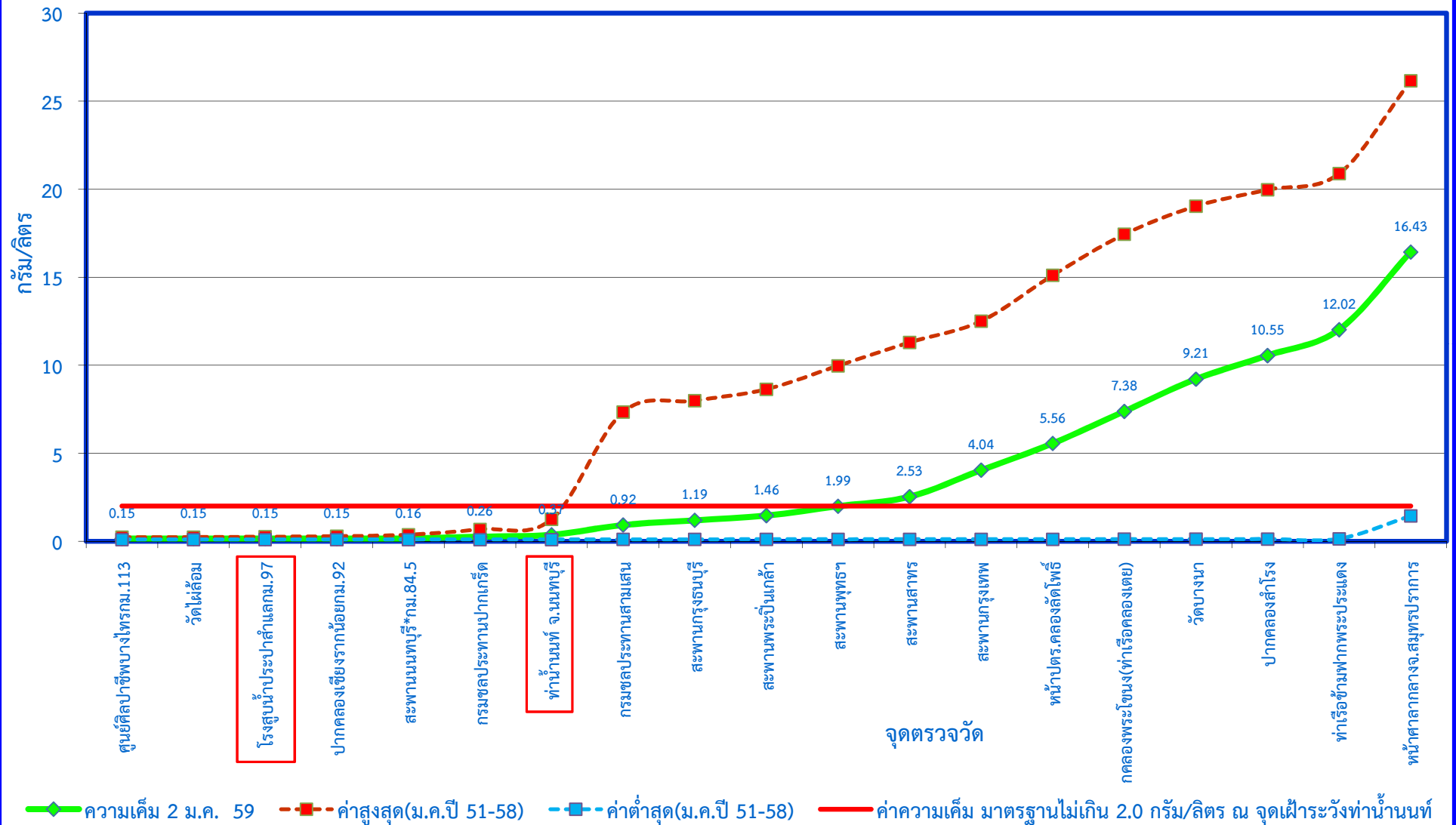
กราฟแสดงค่าความเค็มในแม่น้ำเจ้าพระยาตามพระราชเสาวนีย์ฯ เมื่อวันที่ 2 มกราคม 2559
